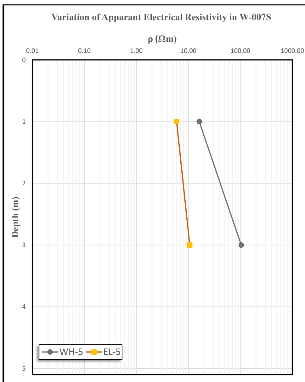
شکل ۳-۷- تغییرات مقاومت الکتریکی بر حسب عمق در موقعیت بسته ی W-007S
