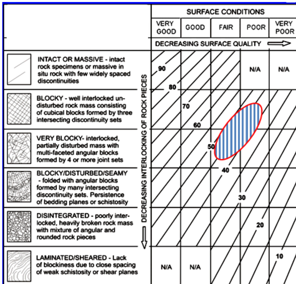
تصویر ۳۹ : شاخص مقاومت زمین شناسی لایه های سیلتستون چاه نفتی W-008N
