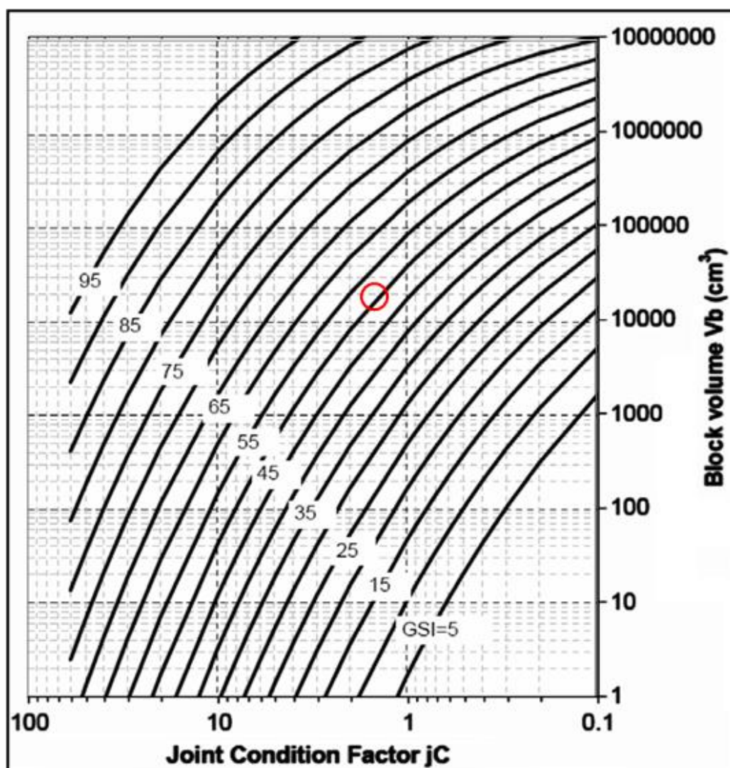
تصویر ۴۲: برآورد کمی GSI لایه های سیلتستون چاه نفتی W-008N به روش Russo, 2009
