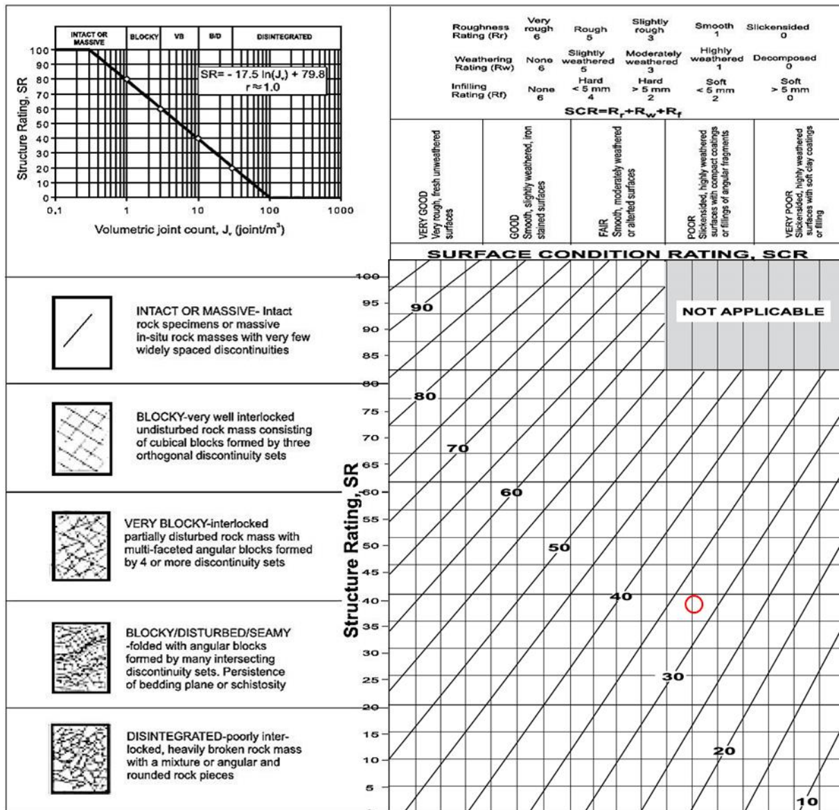
تصویر ۳۵: برآورد کمی GSI لایه های مارنی چاه نفتی W-008N به روش Sonmez & Ulusay, 2002
