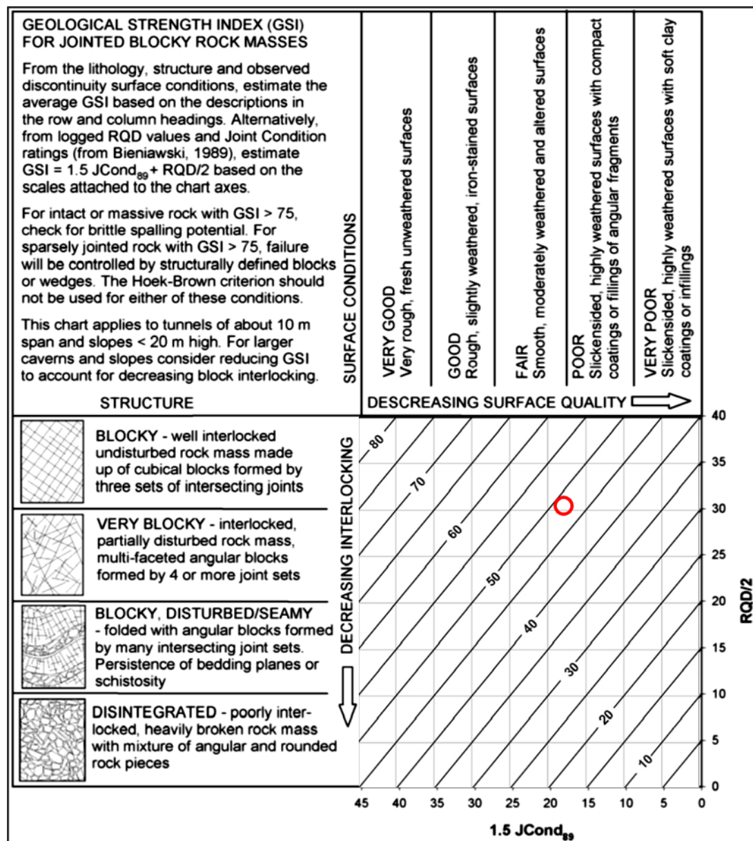
تصویر ۳۸: برآورد کمی GSI لایه های مارنی چاه نفتی W-008N به روش Hoek et al, 2013
