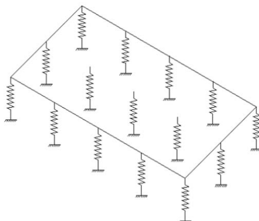
شکل ۶-۱. مدلسازی فنر وینکلر
