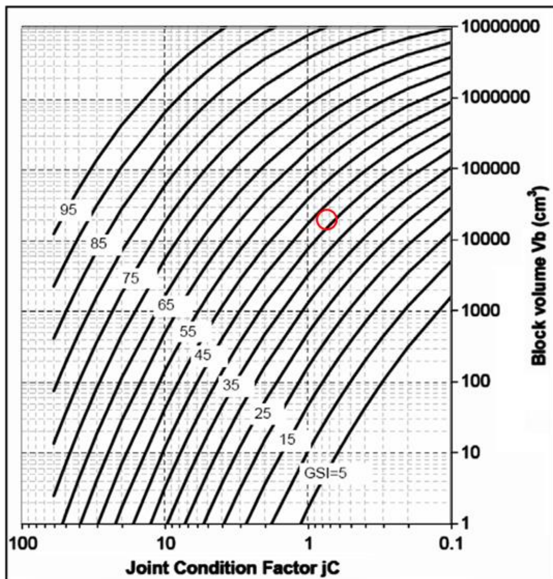
تصویر ۳۷: برآورد کمی GSI لایه های مارنی چاه نفتی W-008N به روش Russo, 2009
