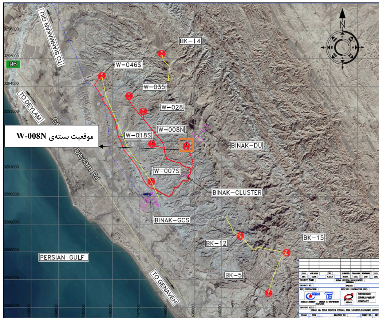
شکل ۲-۱- موقعیت بسته‌ی W-008N نسبت به کل پروژه در Google Earth- نقشه ارسالی از کارفرمای محترم
