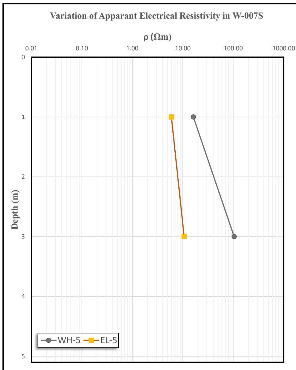
شکل ۳-۷- تغییرات مقاومت الکتریکی بر حسب عمق در موقعیت بسته ی W-007S
