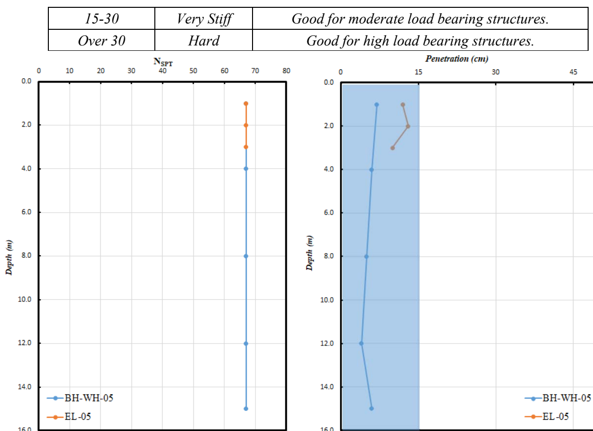
شکل ۳-۴- تغییرات نتایج ضربات SPT (اصلاح نشده) و میزان نفوذ متناظر برحسب عمق موقعیت بسته‌ی W-007S
