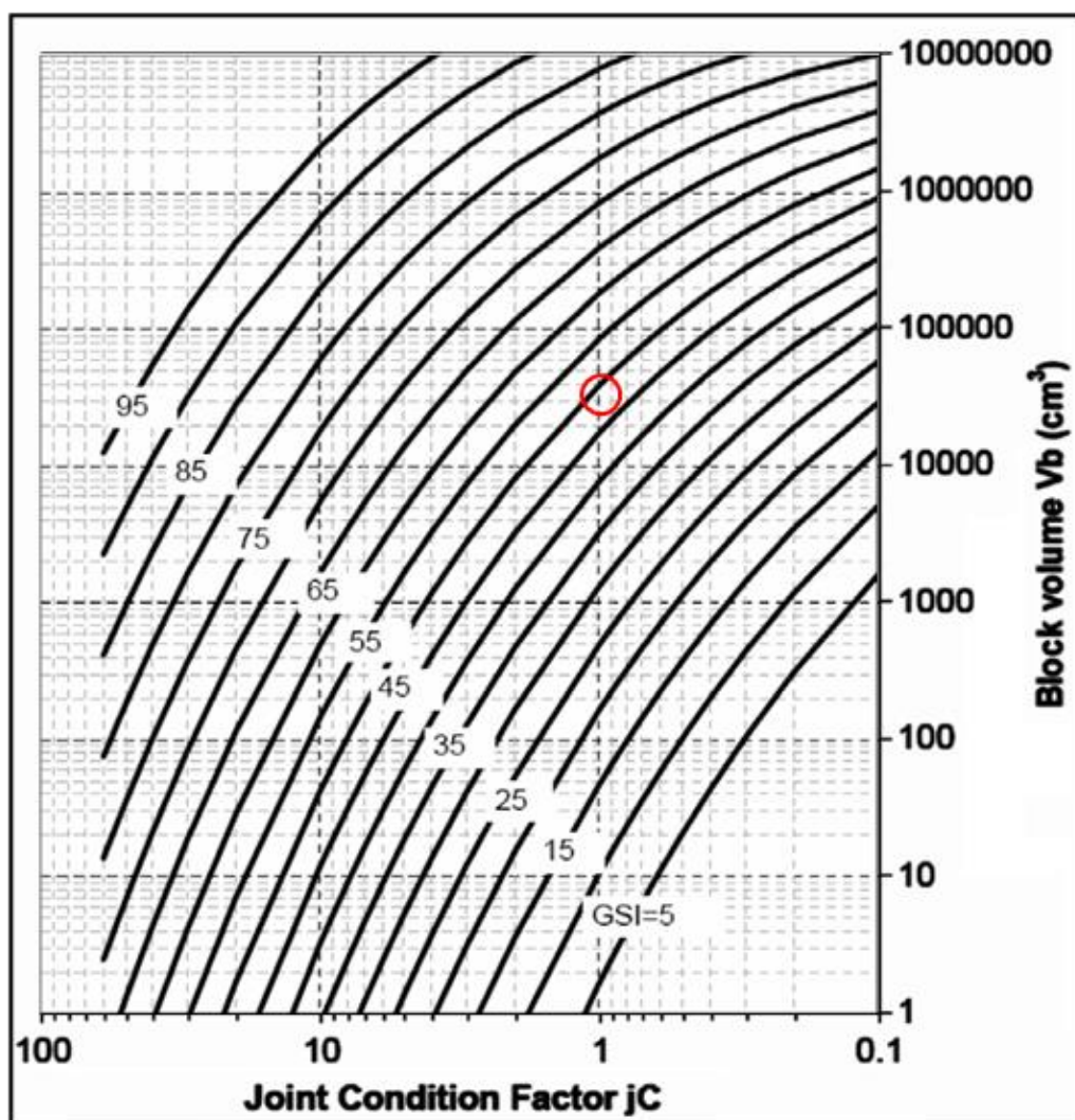
تصویر ۲۶: برآورد کمی GSI لایه های مارنی چاه نفتی BK-07 به روش Russo, 2009
