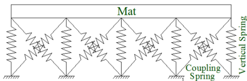
شکل ۶-۲. مدل سازی فنرهای کوپله
