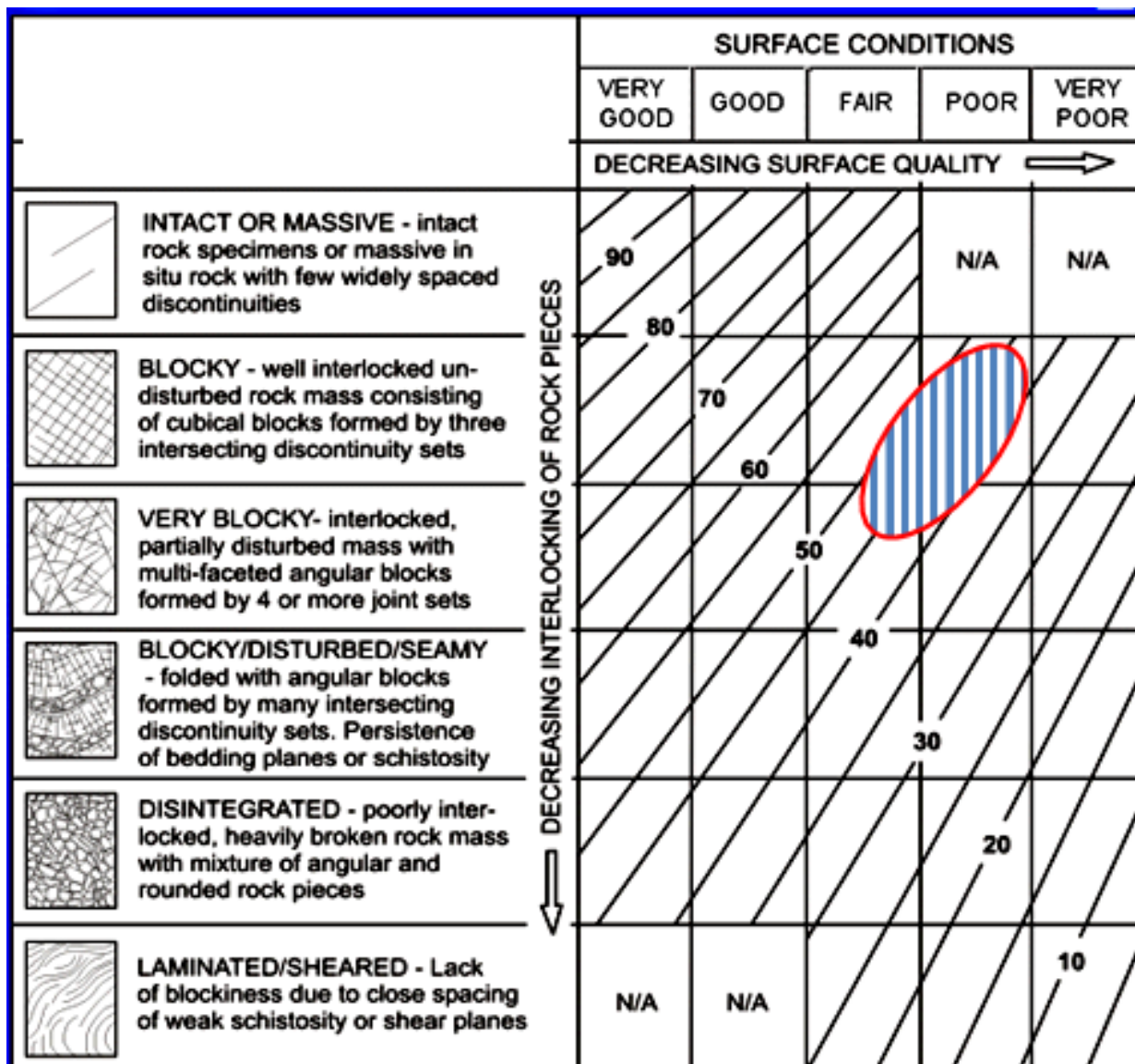
تصویر ۲۳ : شاخص مقاومت زمین شناسی توده سنگ مارنی چاه نفتی BK-07
