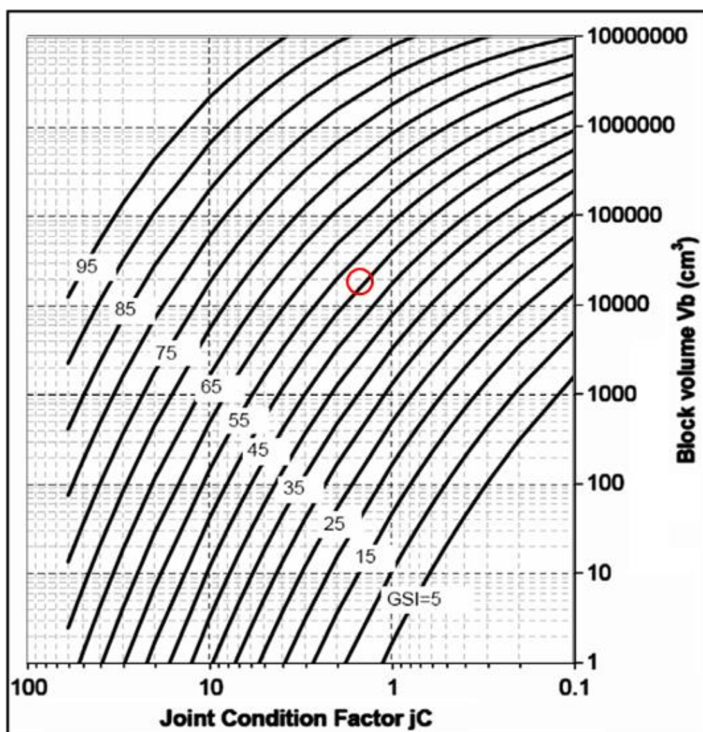
تصویر ۳۱: برآورد کمی GSI لایه های سیلتستون چاه نفتی BK-07 به روش Russo, 2009
