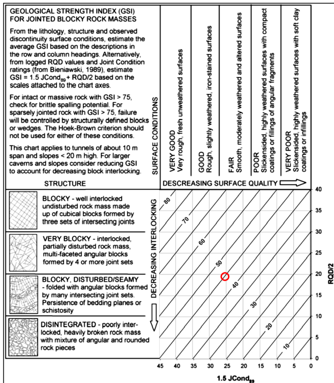
تصویر ۳۲: برآورد کمی GSI لایه های سیلتستون چاه نفتی BK-07 به روش Hoek et al, 2013
