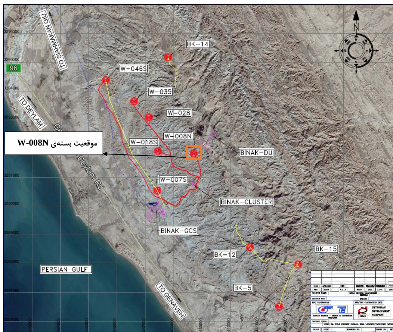
شکل 2-1- موقعیت بسته ی W-008N نسبت به کل پروژه در Google Earth- نقشه ارسالی از کارفرمای محترم
