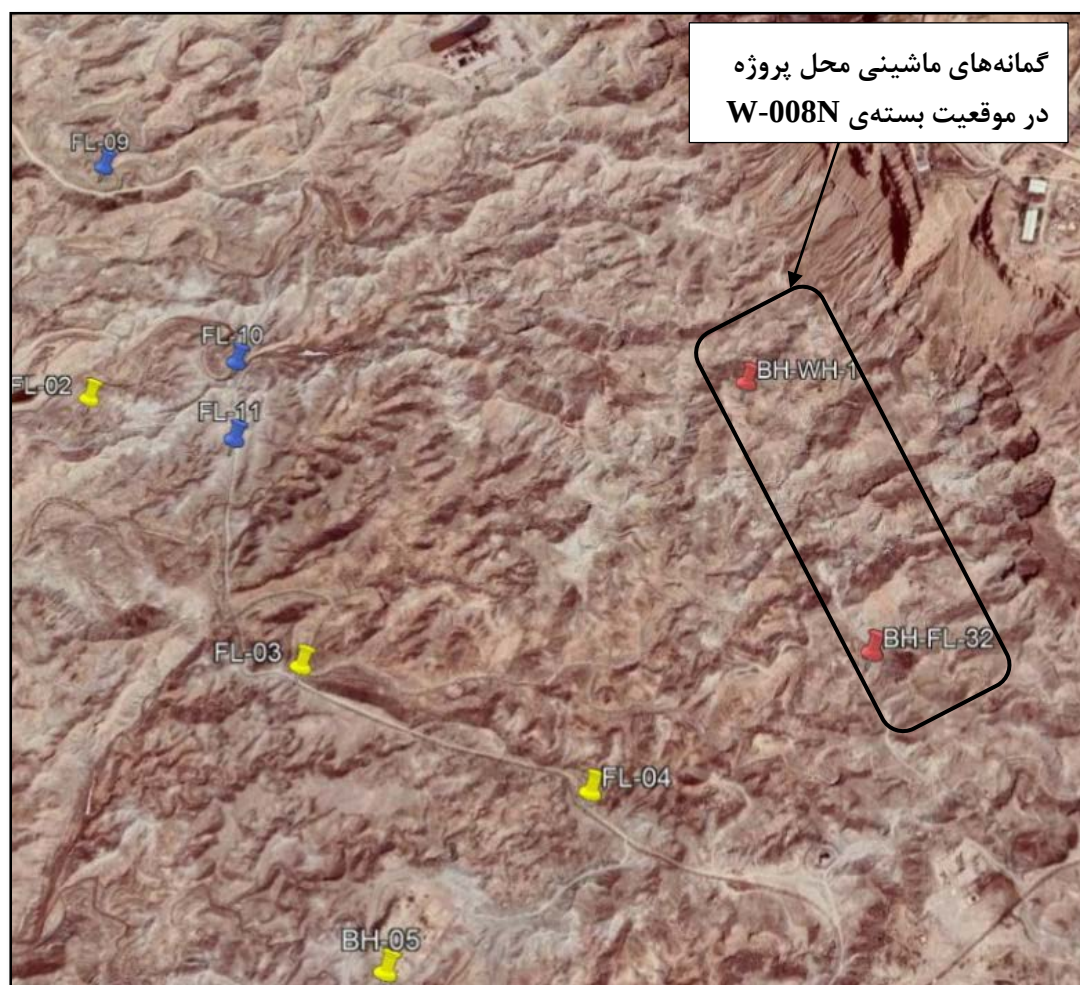
شکل 3-1- جانمایی محل حفر گمانه های ماشینی در موقعیت بسته W-008N نسبت به گمانه های ماشینی مجاور موقعیت مورد نظر در نقشه Google Earth
