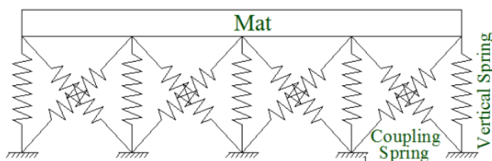
شکل 6-2. مدل سازی فنرهای کوپله
