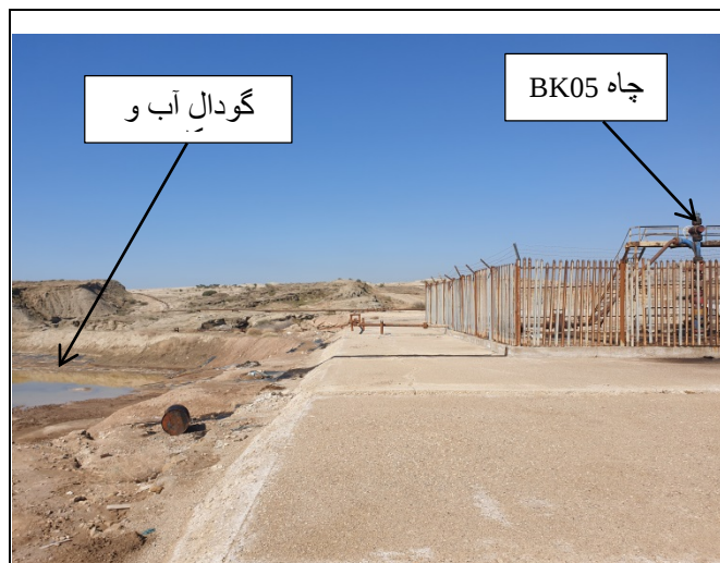
موقعیت گودال نسبت به چاه BK05
