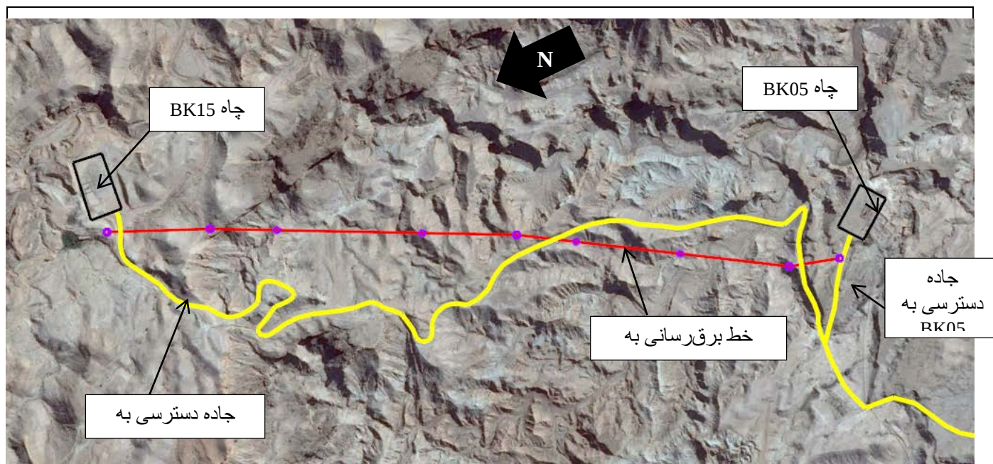
مسیر برق رسانی چاه BK05
