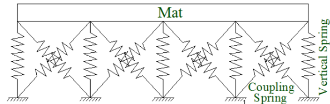
شکل ۶-۲- مدل سازی فنرهای کوپله
