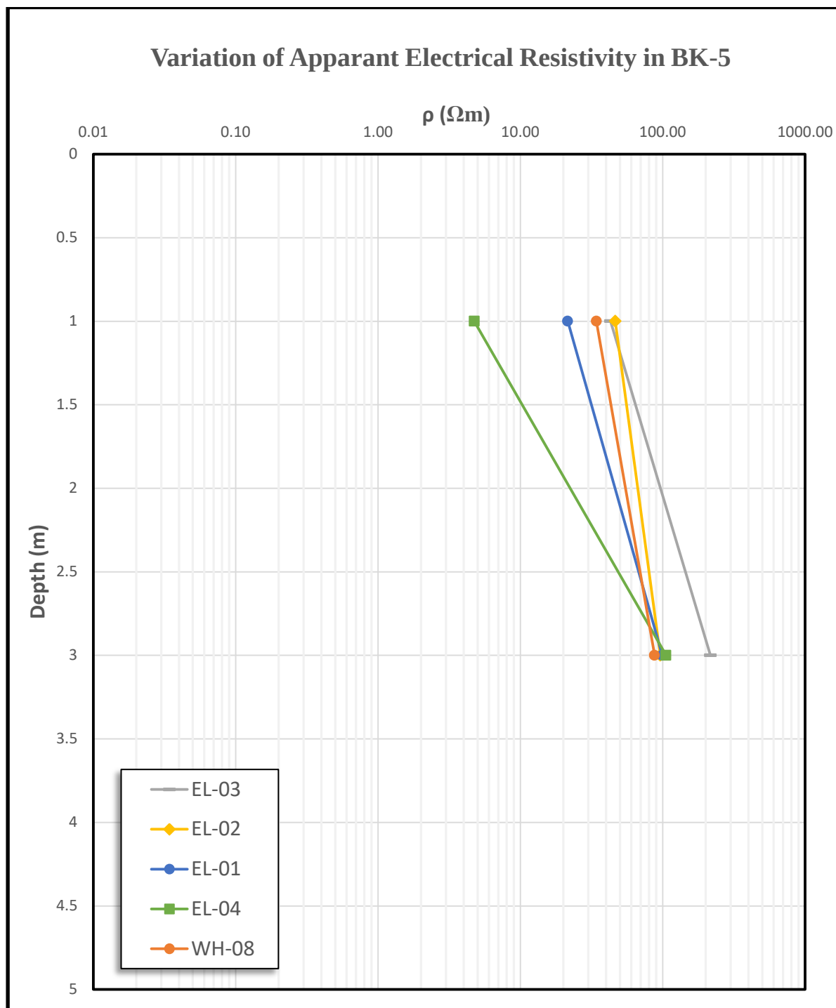
شکل ۳-۶- تغییرات مقاومت الکتریکی بر حسب عمق در بسته ی BK-05
