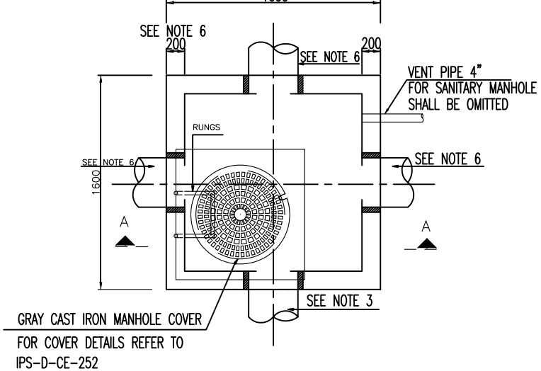
N.T.S 3 MANHOLE PLAN
