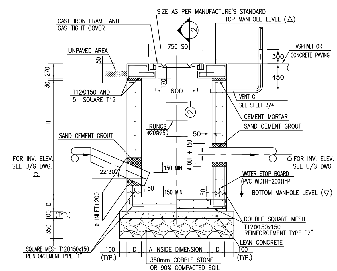
N.T.S 1 MANHOLE FOR ALL AREAS
