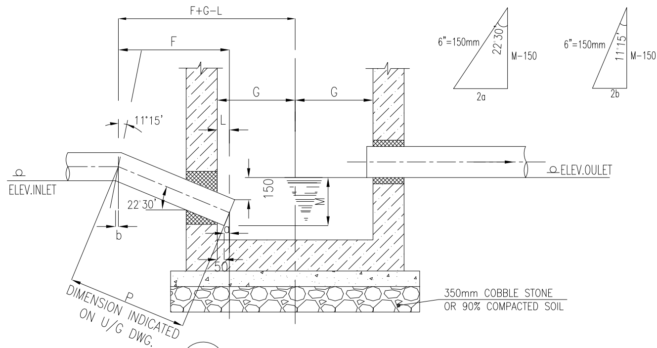
N.T.S 1 MANHOLE DIMENSION
