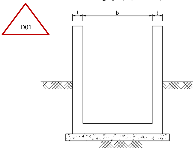
طرح شماتیک کانال بتنی
