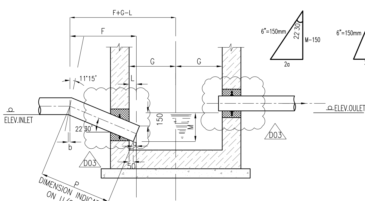
N.T.S 1 MANHOLE DIMENSION
