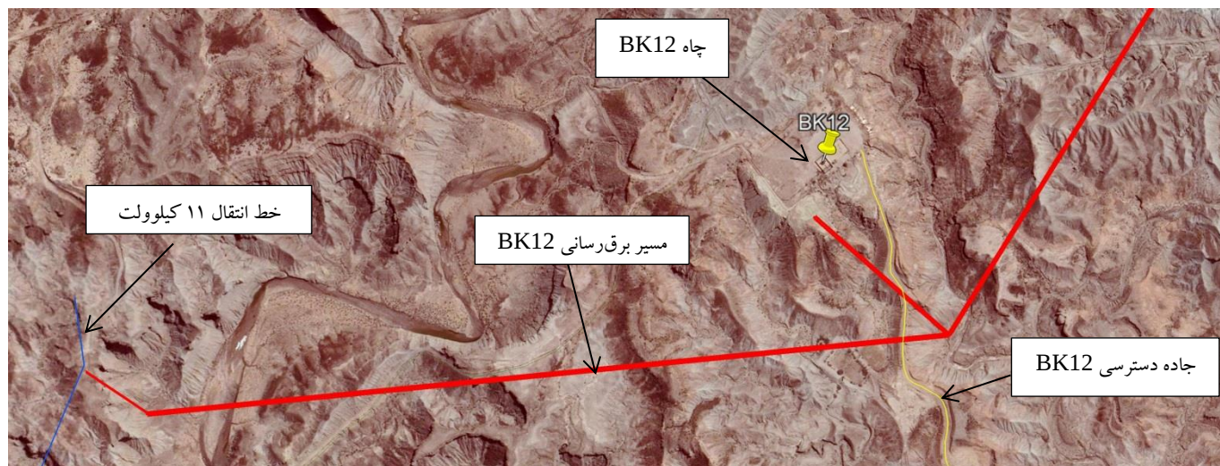
مسیر برق رسانی چاه BK12
