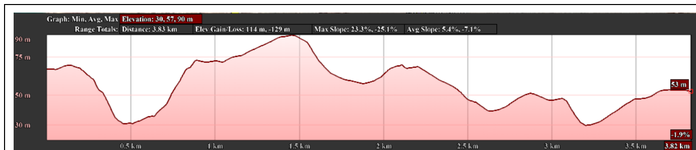
پروفیل طولی خط لوله جریانی از چاه BK12 تا کلاستر بینک (استخراج شده از Google Earth)
