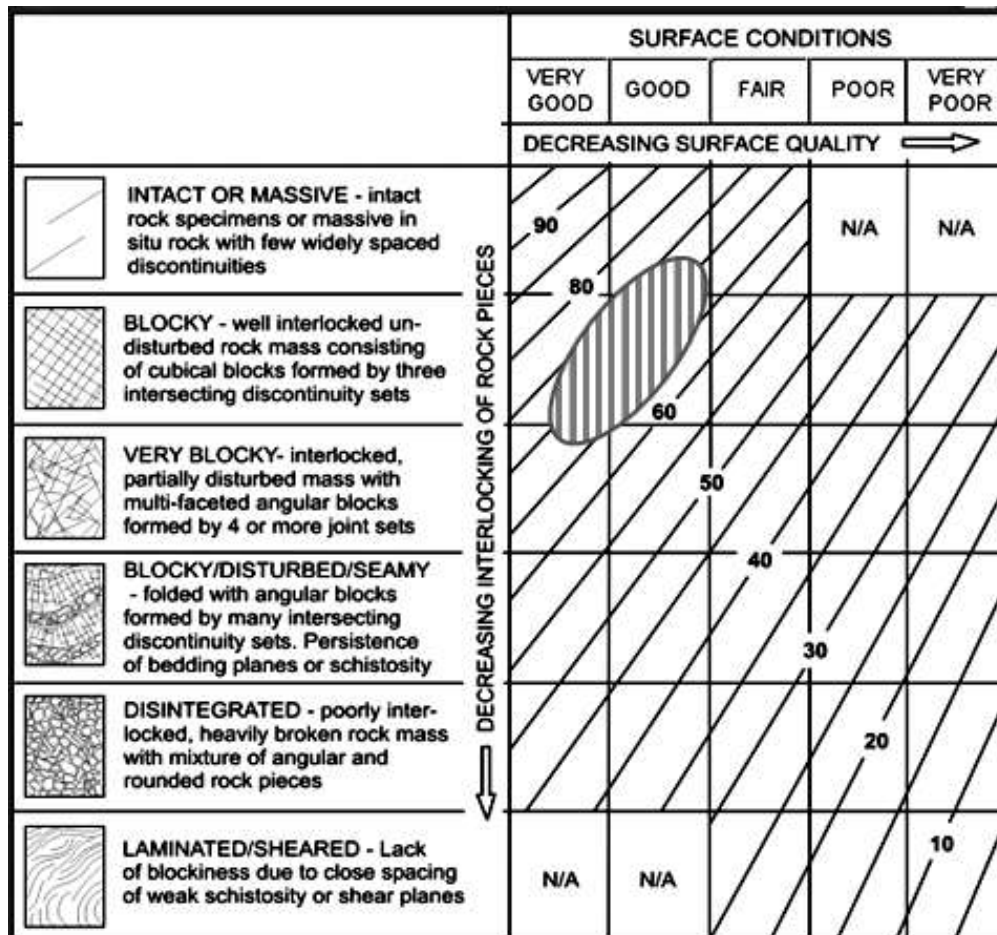
تصویر ۱۷ : شاخص مقاومت زمین شناسی لایه های ماسه سنگ چاه نفتی BK-14
