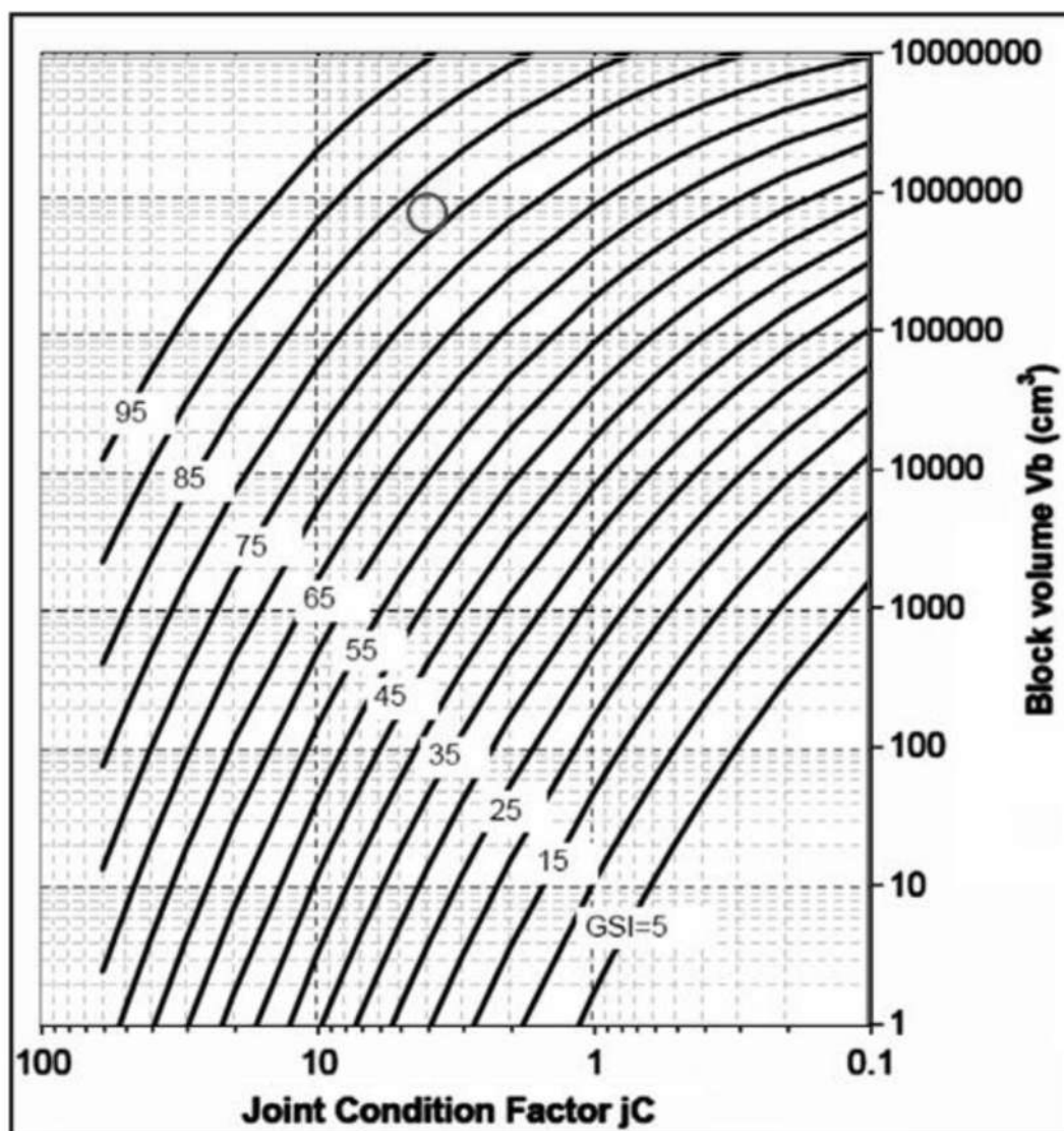
تصویر ۲۰: برآورد کمی GSI لایه های ماسه سنگ چاه نفتی BK-14 به روش Russo, 2009
