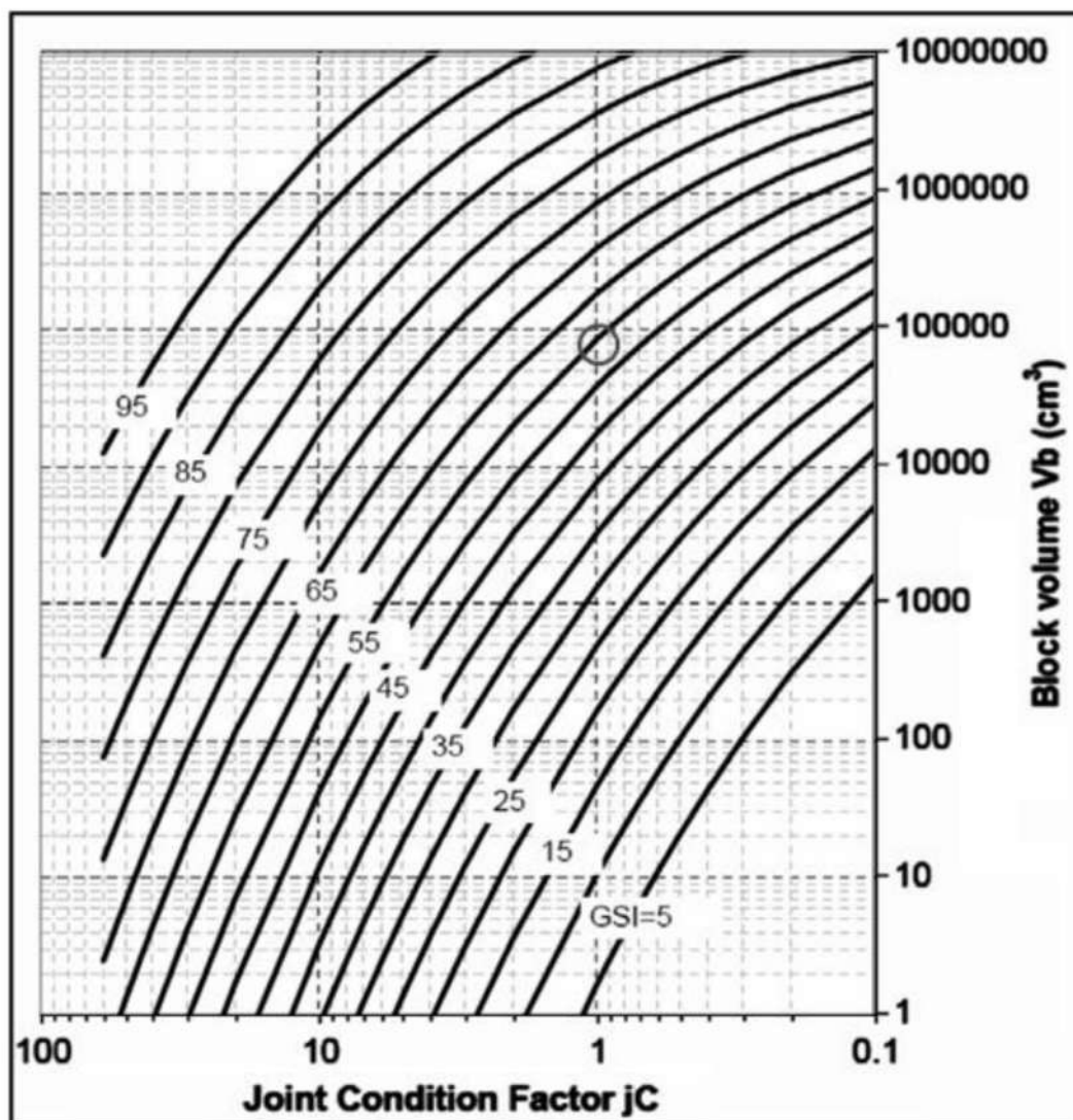
تصویر ۱۵: برآورد کمی GSI لایه های مارنی چاه نفتی BK-14 به روش Russo, 2009
