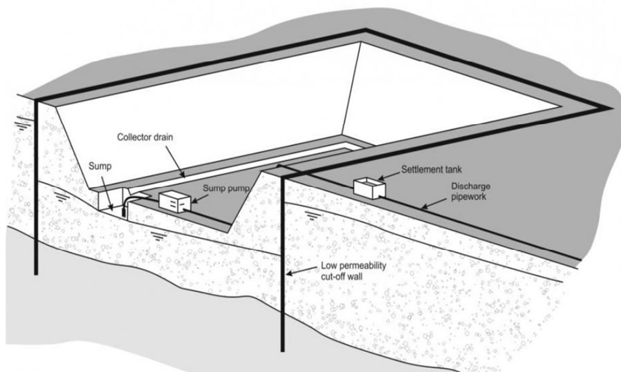
شکل 3-7 - روش نهر و پمپاژ از گودال
