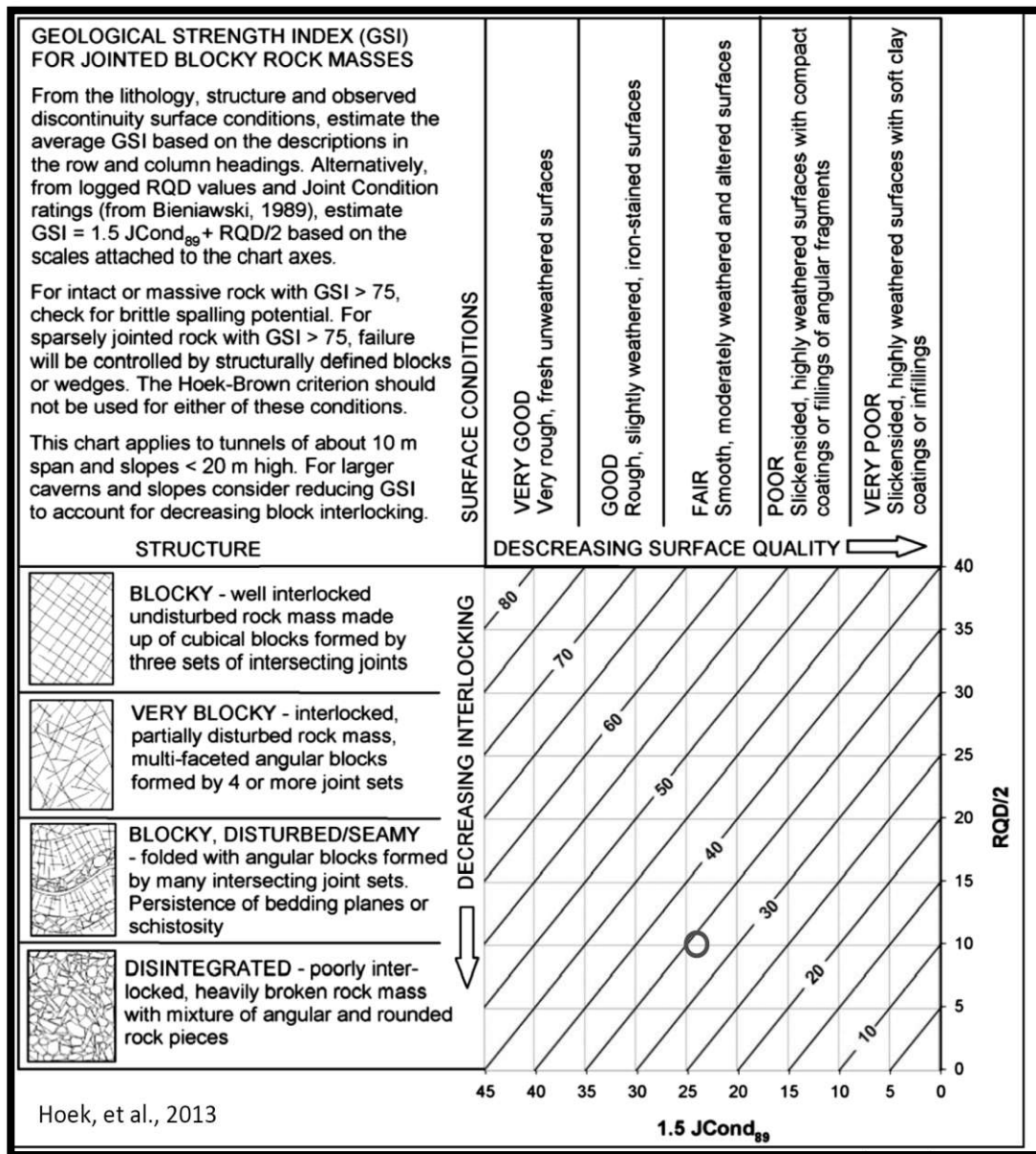
تصویر ۱۰: برآورد کمی GSI به روش Hoek et al, 20
