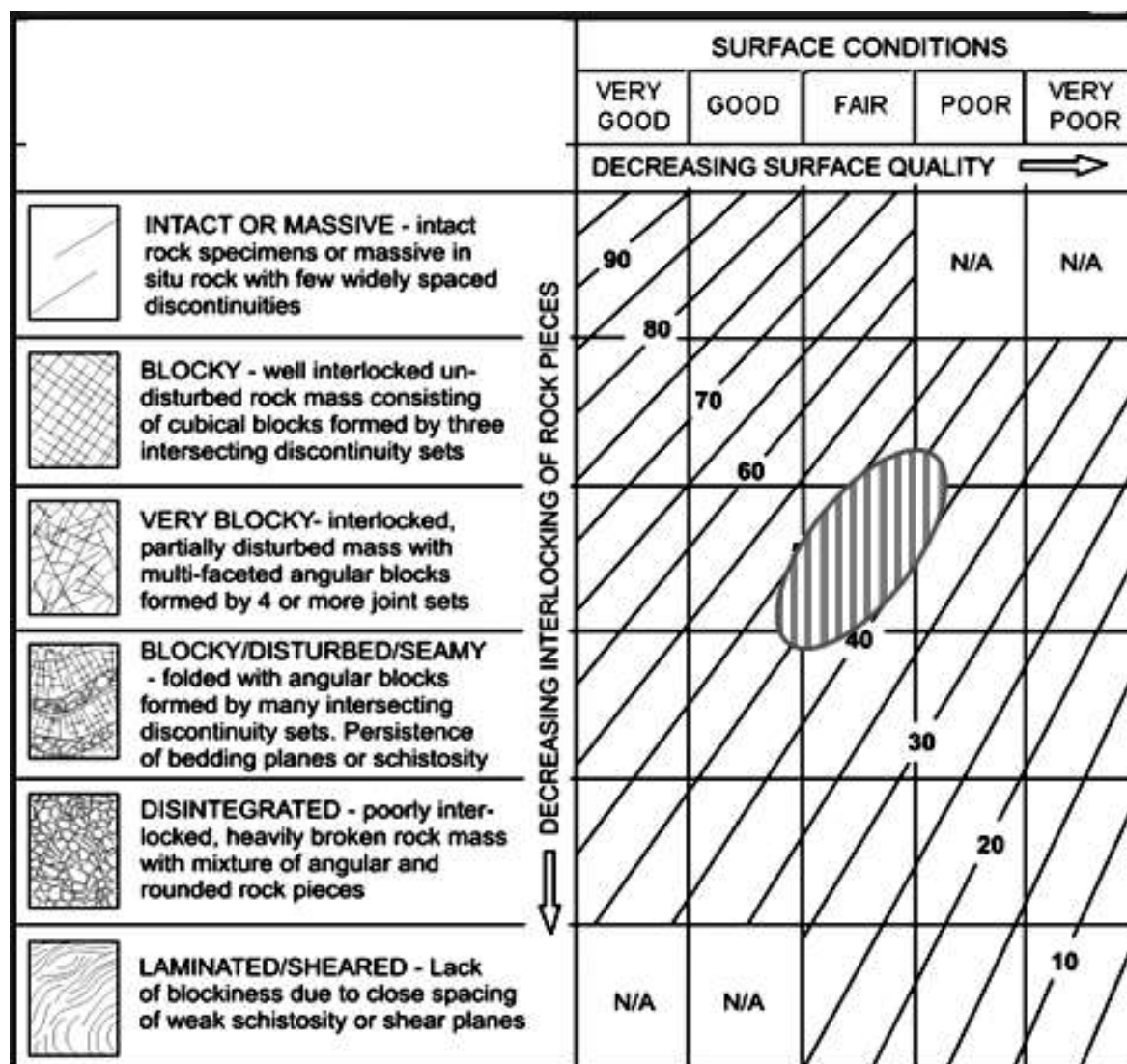
تصویر ۱۲: شاخص مقاومت زمین شناسی توده سنگ مارنی چاه نفتی BK-14
