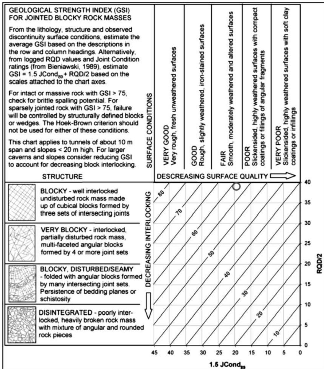
تصویر ۱۶: برآورد کمی GSI لایه های مارنی چاه نفتی BK-14 به روش Hoek et al, 2013
