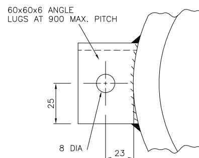
TYPE 'B' RING
