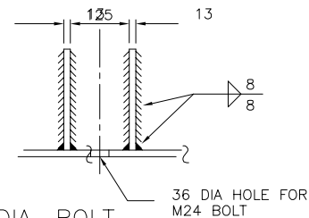
TYPE 1- BASE LUG FOR M24 DIA. BOLT
