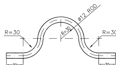
DETAIL 3 LUG (HANDLE)
