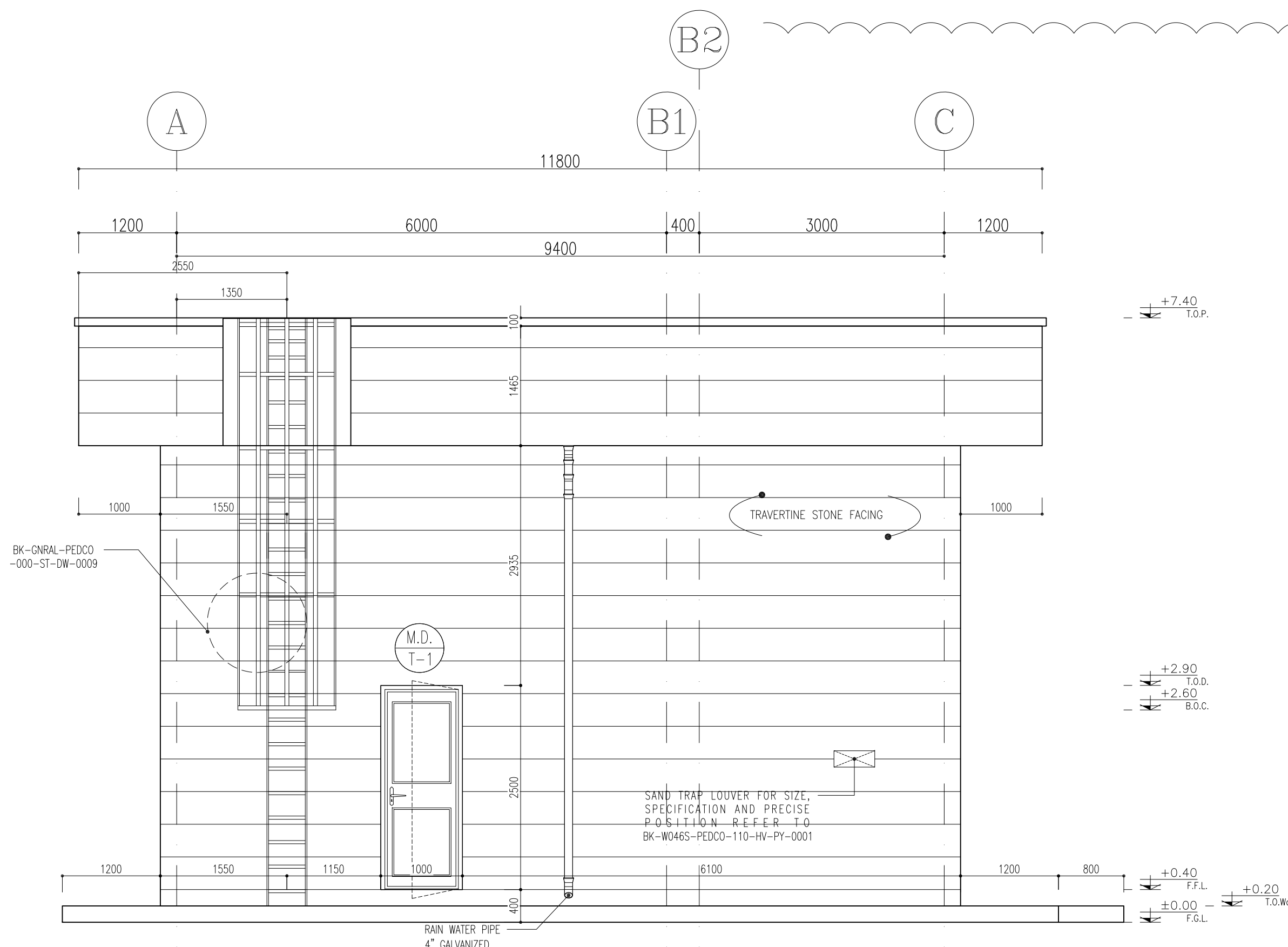
SC.1:50 1 ELEVATION
