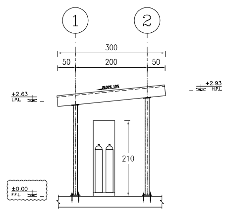
2 ELEVATION SC. 1:50
