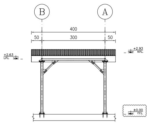
3 ELEVATION SC. 1:50
