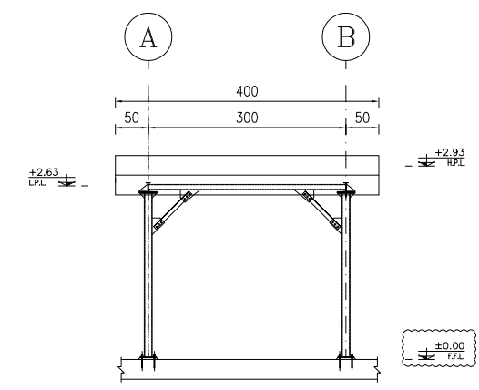
4 ELEVATION SC. 1:50
