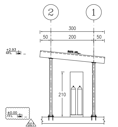
1 ELEVATION SC. 1:50
