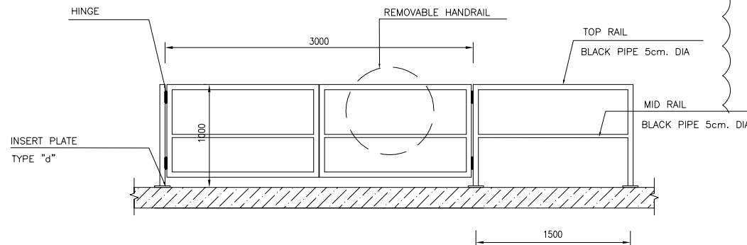
07 DETAIL 07 SC:1:25
