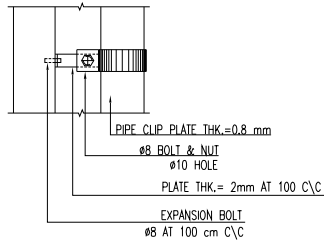
02 DETAIL 02 SC:1:10
