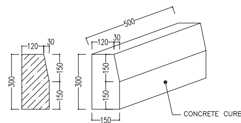
07 DETAIL 07 SC:1:25
