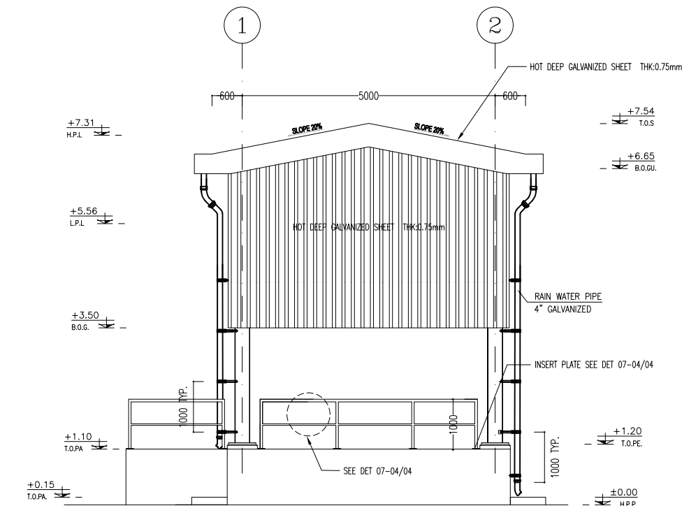
3 ELEVATION
