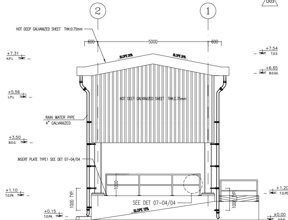
2 ELEVATION
