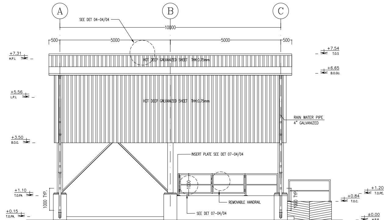
1 ELEVATION
