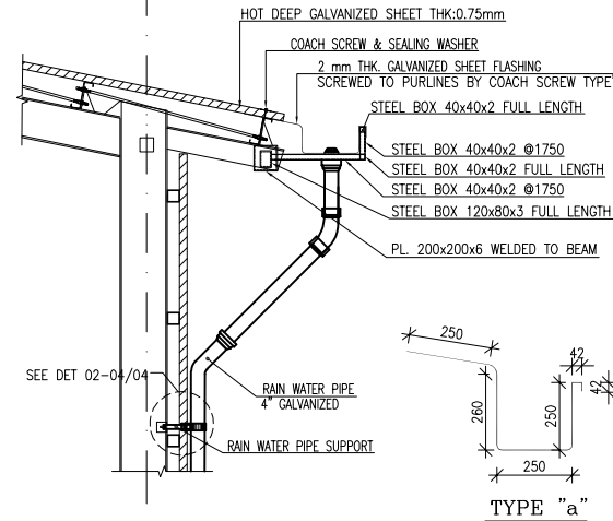
06 DETAIL 06 SC:1:25
