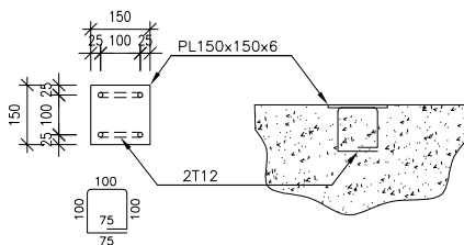
08 DETAIL 08 SC:1:10
