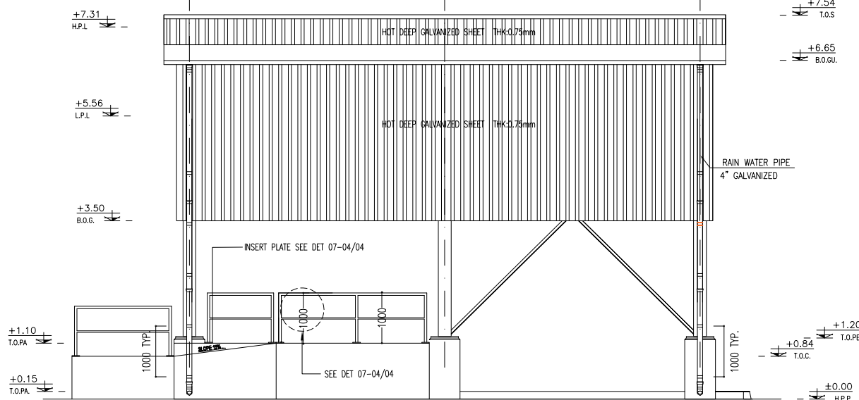
4 ELEVATION
