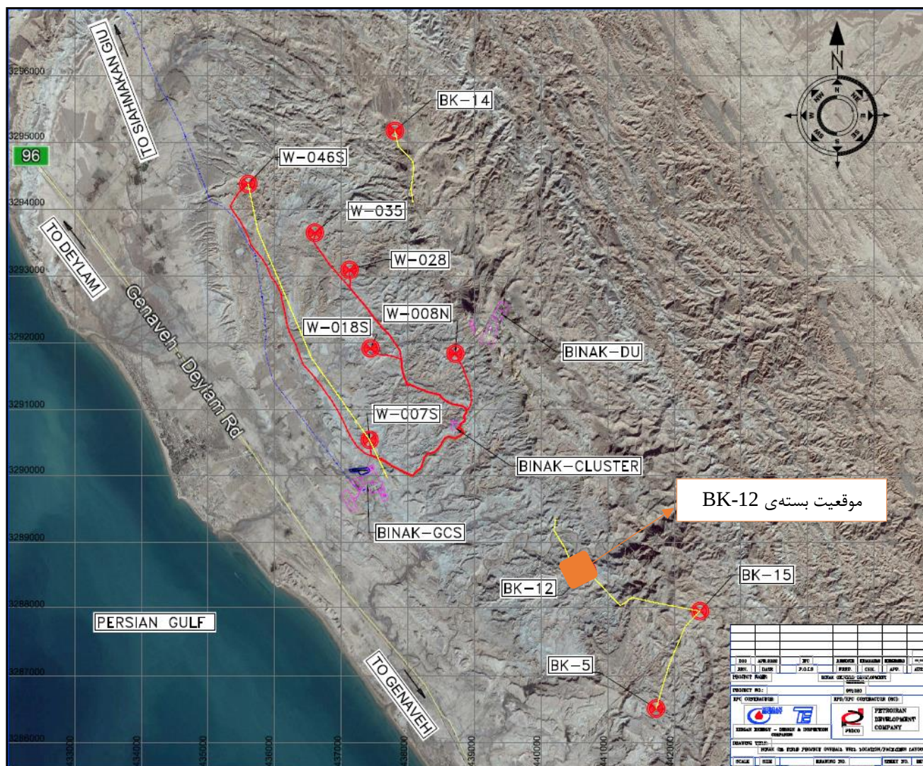
شکل ۳-۳- موقعیت بسته ی BK-12 نسبت به مسیر خط لوله نقشه ارسالی از شرکت محترم هیرگان انرژی
