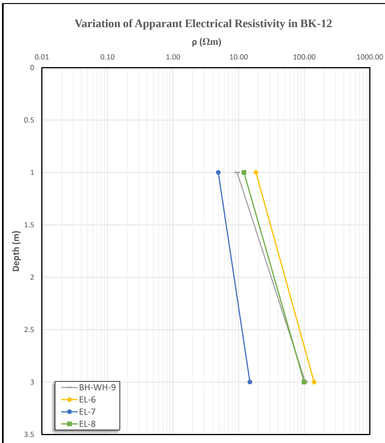
شکل ۳-۶- تغییرات مقاومت الکتریکی بر حسب عمق در بسته ی BK-12
