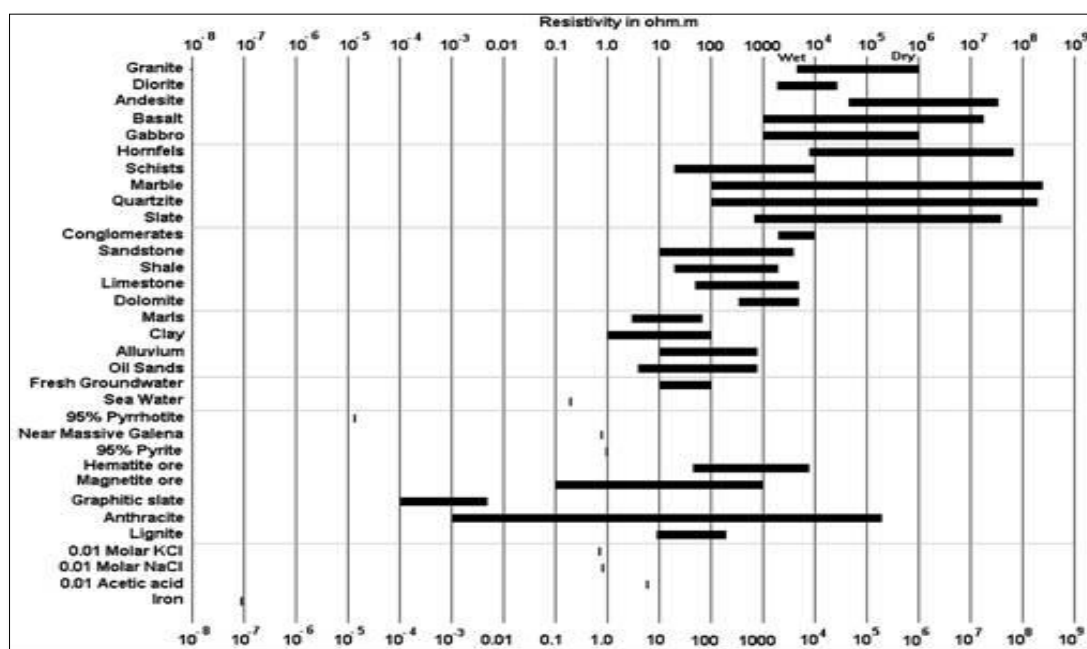
شکل ۵-۳- حدود مقاومت الکتریکی برای خاک های مختلف
