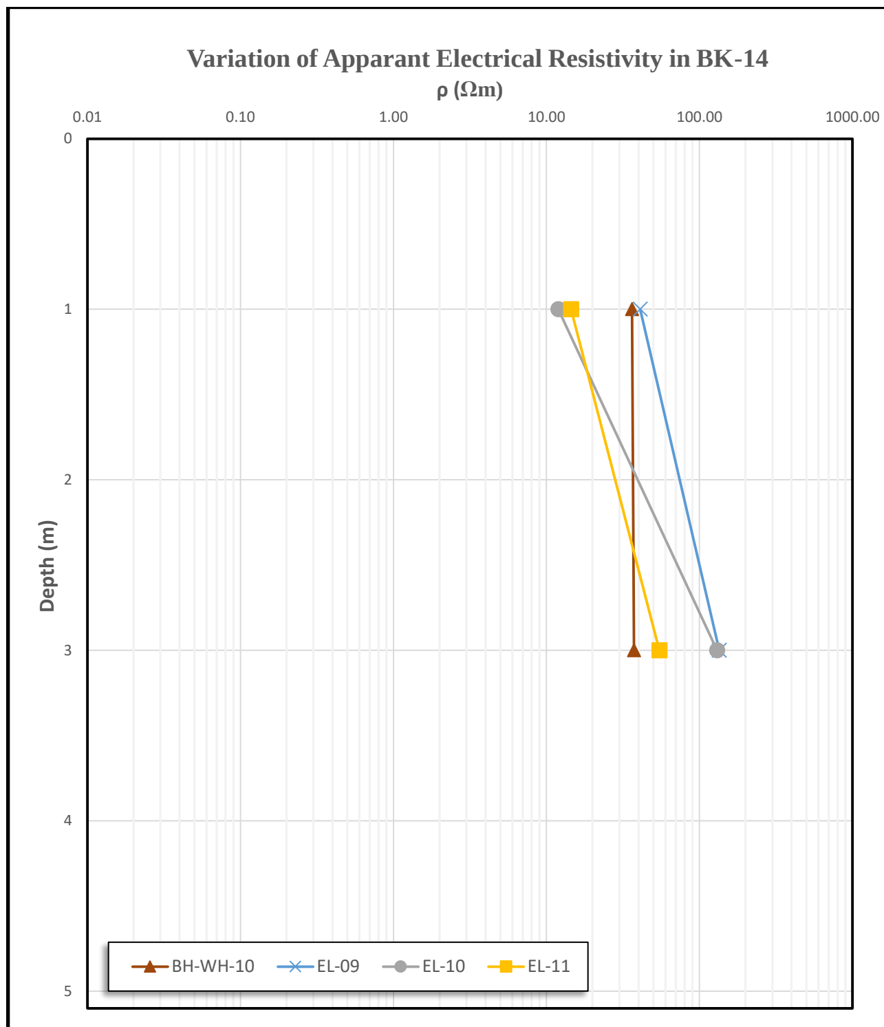
شکل ۳-۵- تغییرات مقاومت الکتریکی بر حسب عمق در بسته ی BK-14
