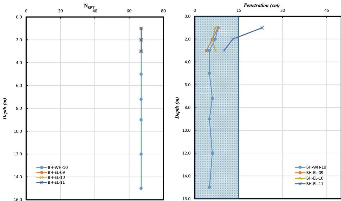
شکل ۳-۳- تغییرات نتایج ضربات SPT (اصلاح نشده) و میزان نفوذ متناظر بر حسب عمق بسته‌ی BK-14
