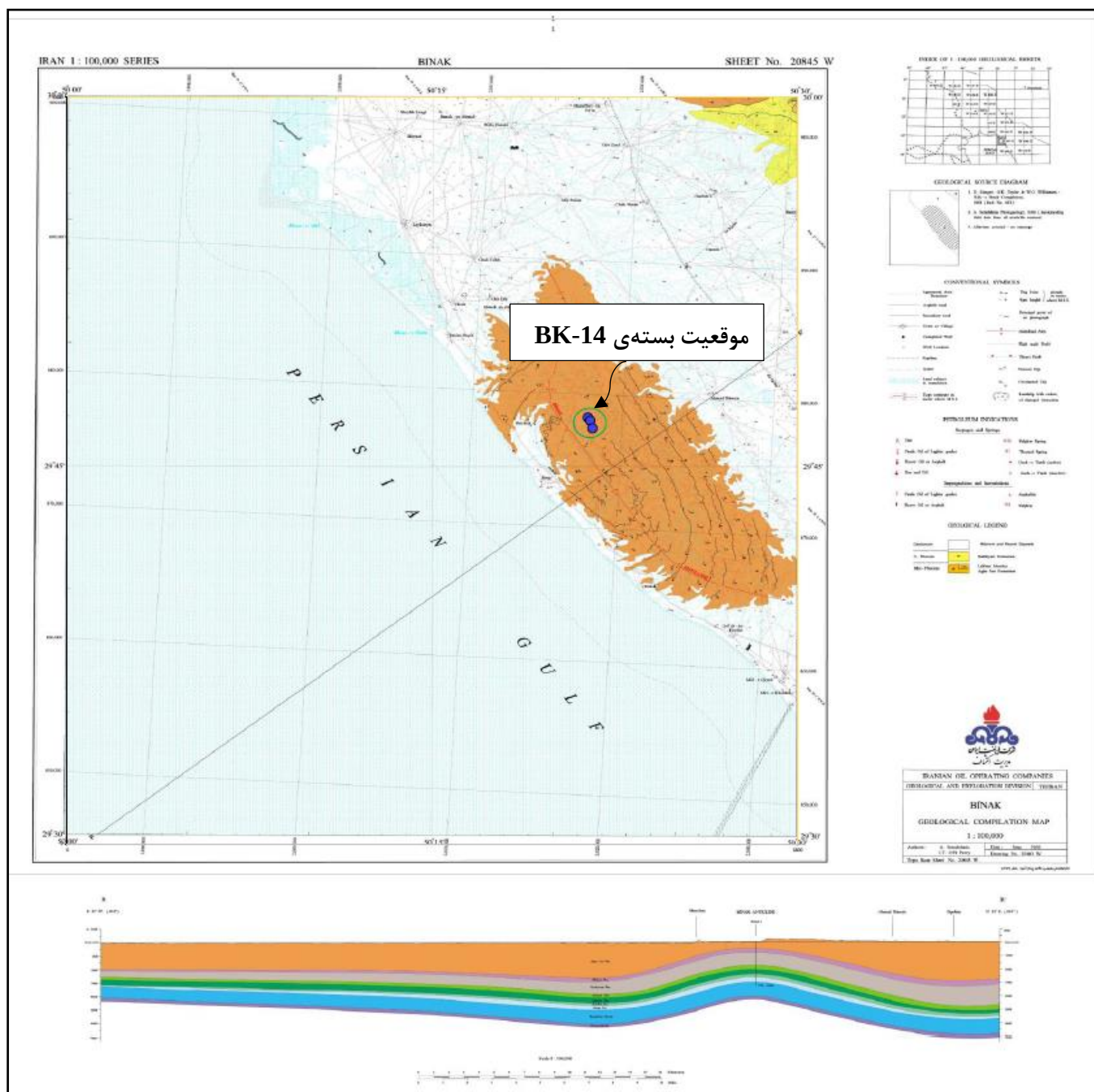
شکل ۲-۴- موقعیت بسته ی BK-14 در نقشه زمین شناسی بوشهر در منطقه بینک به مقیاس ۱:۱۰۰۰۰۰
