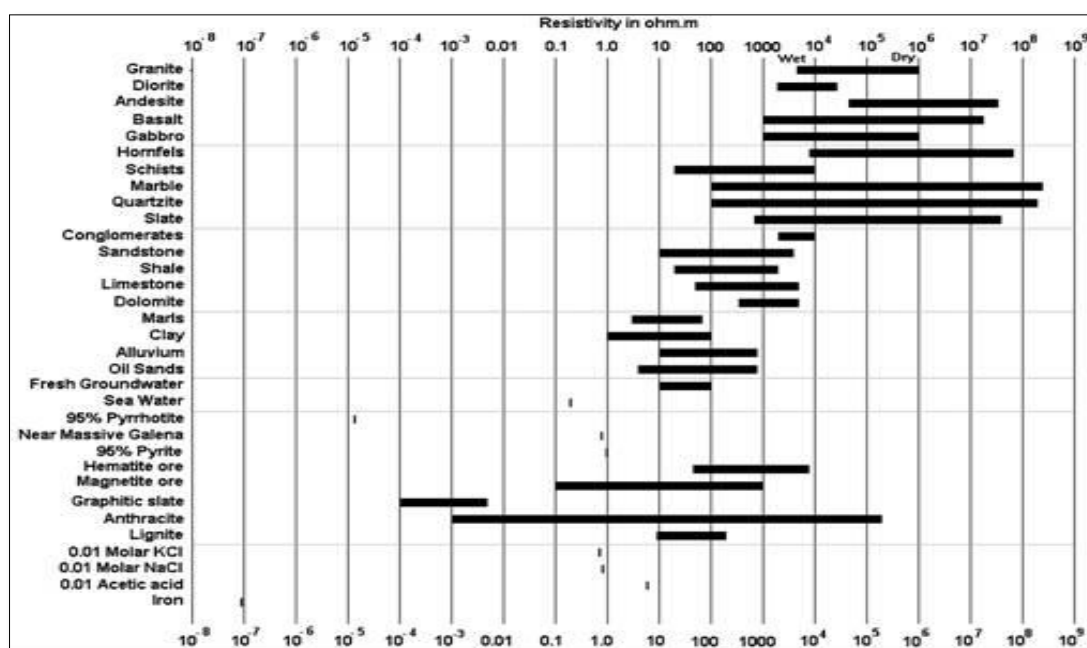
شکل ۳-۴- حدود مقاومت الکتریکی برای خاک های مختلف
