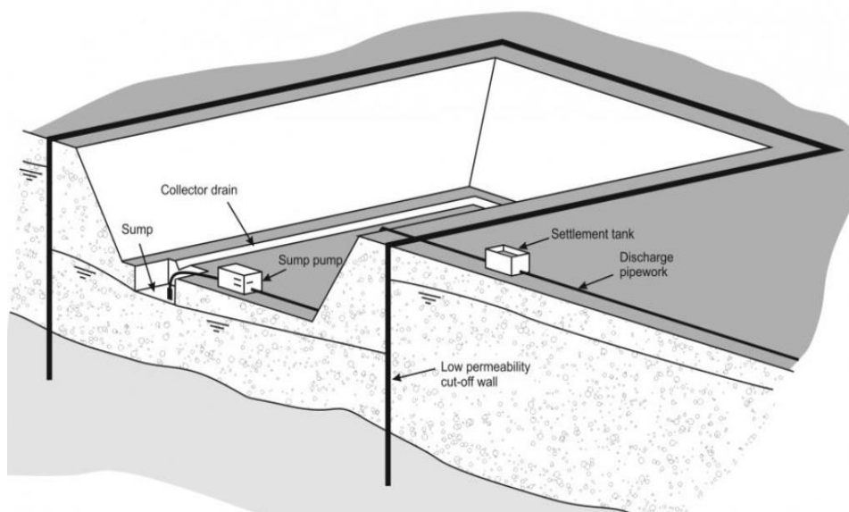
شکل ۷-۳ - روش نهر و پمپاژ از گودال
