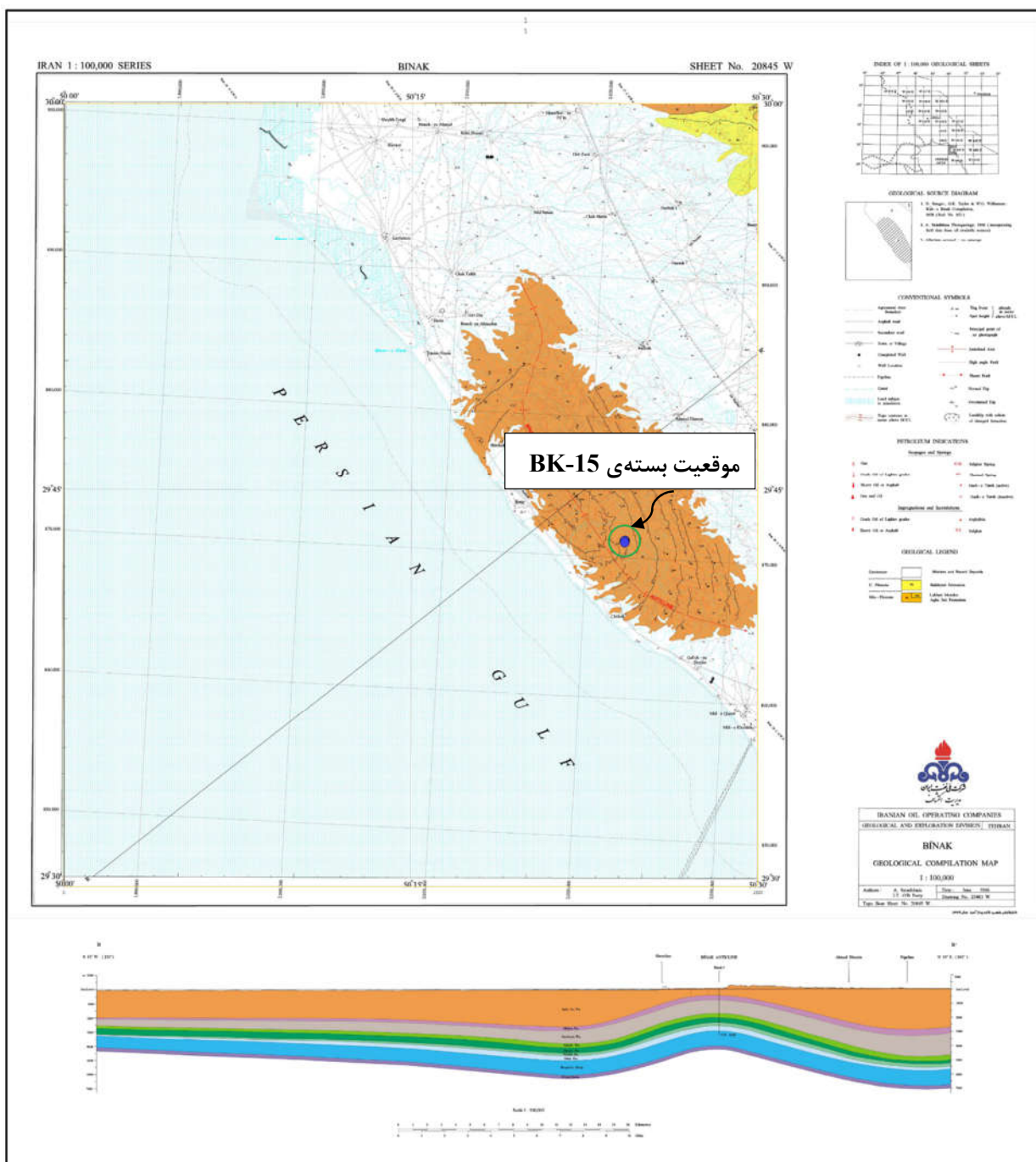
شکل 2-4- موقعیت بسته‌ی BK-15 در نقشه زمین‌شناسی بوشهر در منطقه بینک به مقیاس 1:100000
