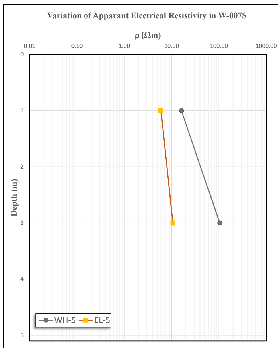
شکل 3-7- تغییرات مقاومت الکتریکی بر حسب عمق در موقعیت بسته ی W-007S
