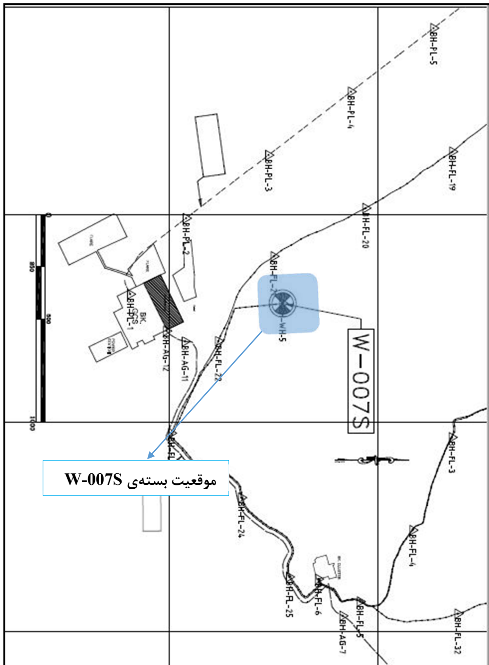
شکل 2-3- موقعیت قرارگیری محل حفر گمانه‌های ماشینی در بسته‌ی W-007S - نقشه ارسالی از کارفرمای محترم
