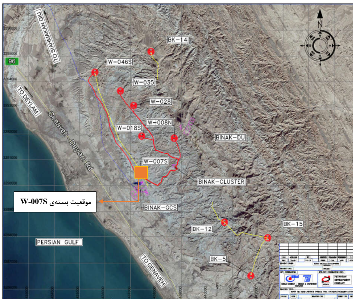
شکل 3-3- موقعیت قرارگیری محل حفر گمانه‌های ماشینی در بسته‌ی W-007S - نقشه ارسالی از کارفرمای محترم
