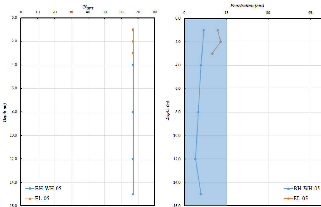
شکل 3-4- تغییرات نتایج ضربات SPT (اصلاح نشده) و میزان نفوذ متناظر برحسب عمق موقعیت بسته‌ی W-007S
