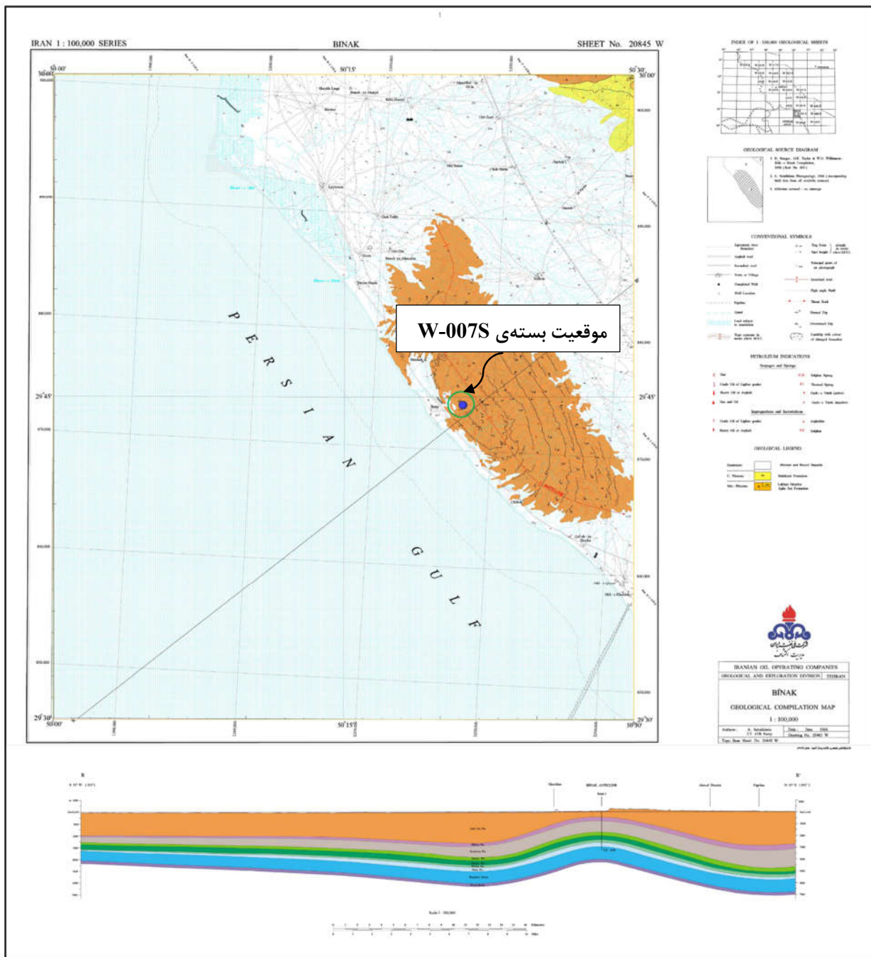
شکل 2-4- موقعیت بسته‌ی W-007S در نقشه زمین‌شناسی بوشهر در منطقه بینک به مقیاس 1:100000
