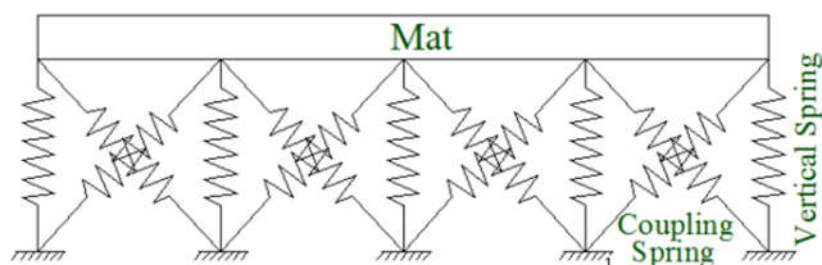
شکل 2-6 مدل سازی فنرهای کوپله
