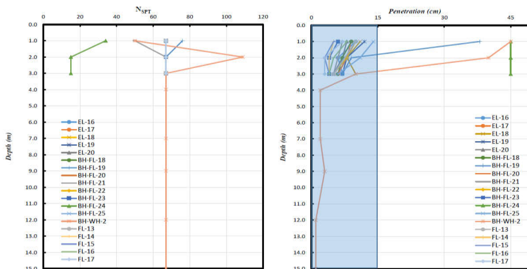
شکل 3-4- تغییرات نتایج ضربات SPT (اصلاح نشده) و میزان نفوذ متناظر برحسب عمق بسته ی W-046
