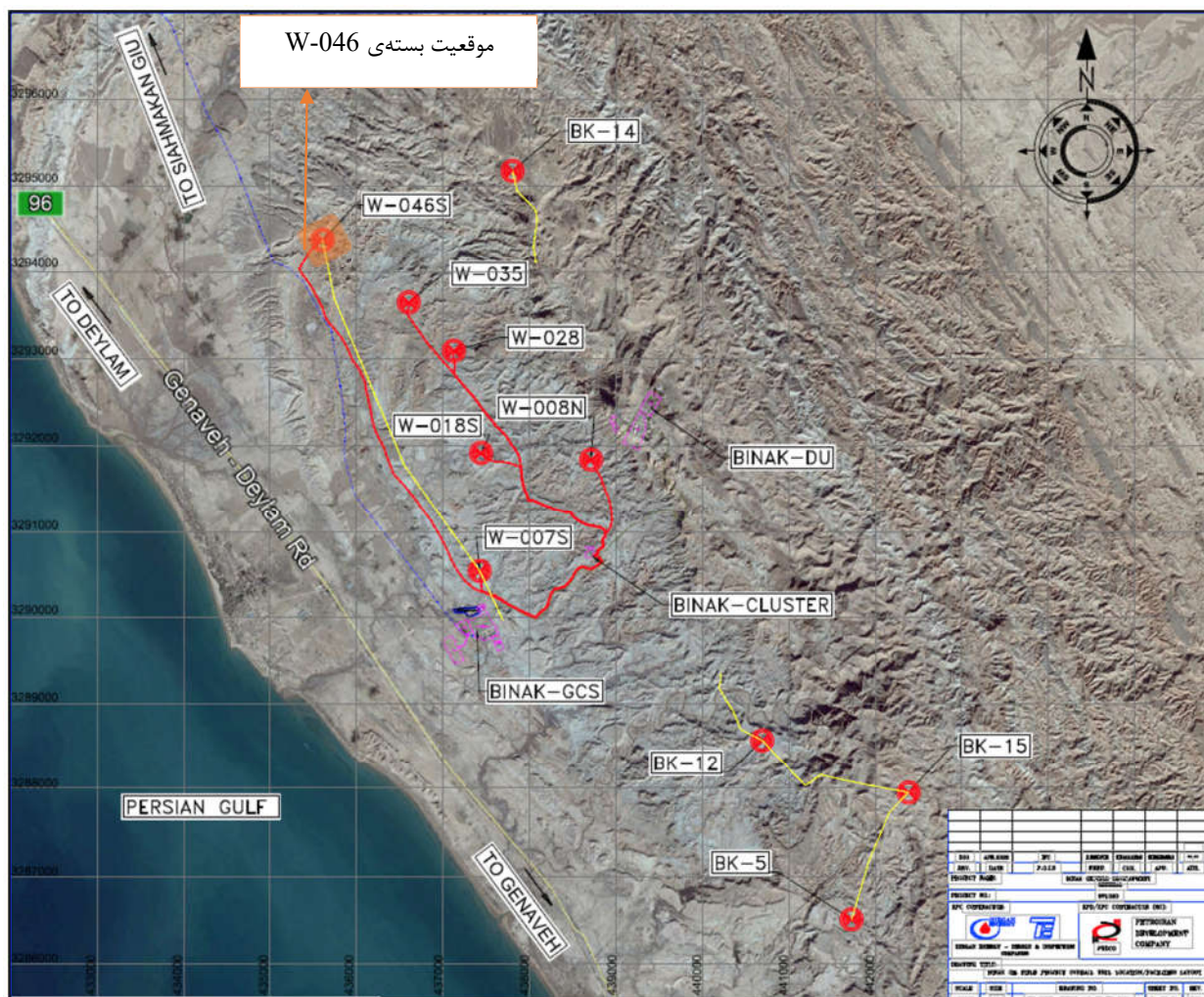
شکل 3-3- موقعیت قرارگیری محل حفر گمانه های ماشینی در موقعیت بسته ی W-046- نقشه ارسالی از شرکت محترم هیرگان انرژی
