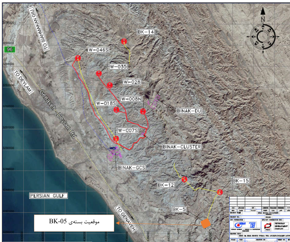
شکل 3-3- موقعیت قرارگیری محل حفر گمانه های ماشینی در موقعیت بسته ی BK-05 - نقشه ارسالی از شرکت محترم هیرگان انرژی جدول 3-1. مشخصات کلی گمانه های ماشینی موقعیت بسته ی BK-05
