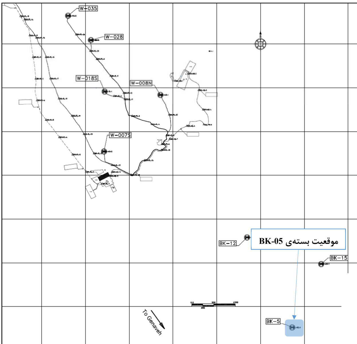
شکل 3-2- جانمایی محل حفر گمانه های ماشینی در موقعیت بسته ی BK-05 نسبت به مسیرهای خط لوله- نقشه ارسالی از شرکت محترم هیروگان انرژی
