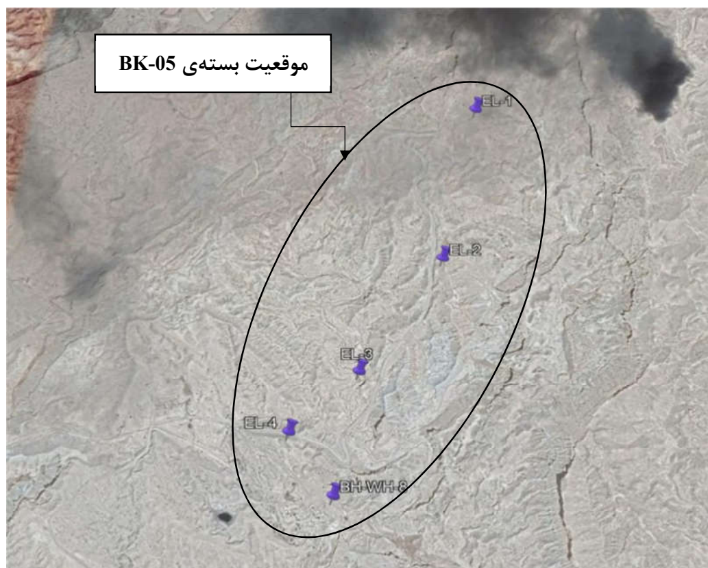
شکل 4-1- گمانه های ماشینی در محدوده مورد مطالعه موقعیت بسته ی BK-05
