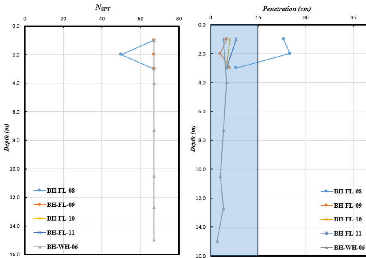
شکل 4-3- تغییرات نتایج ضربات SPT (اصلاح نشده) و میزان نفوذ متناظر برحسب عمق W-028
