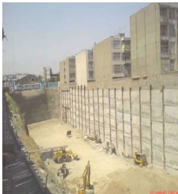
شکل 7-1 - تصاویری از سازه های نگهدارنده جهت گودبرداری (روش نیلینگ و دیوار برلنی)
