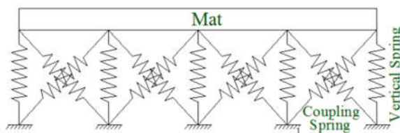
شکل 6-2. مدل سازی فنرهای کوپله
