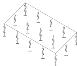
شکل 6-1. مدلسازی فنر وینکلر
