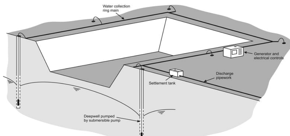
شکل 2-7 - سیستم آبکشی از چاه های عمیق
