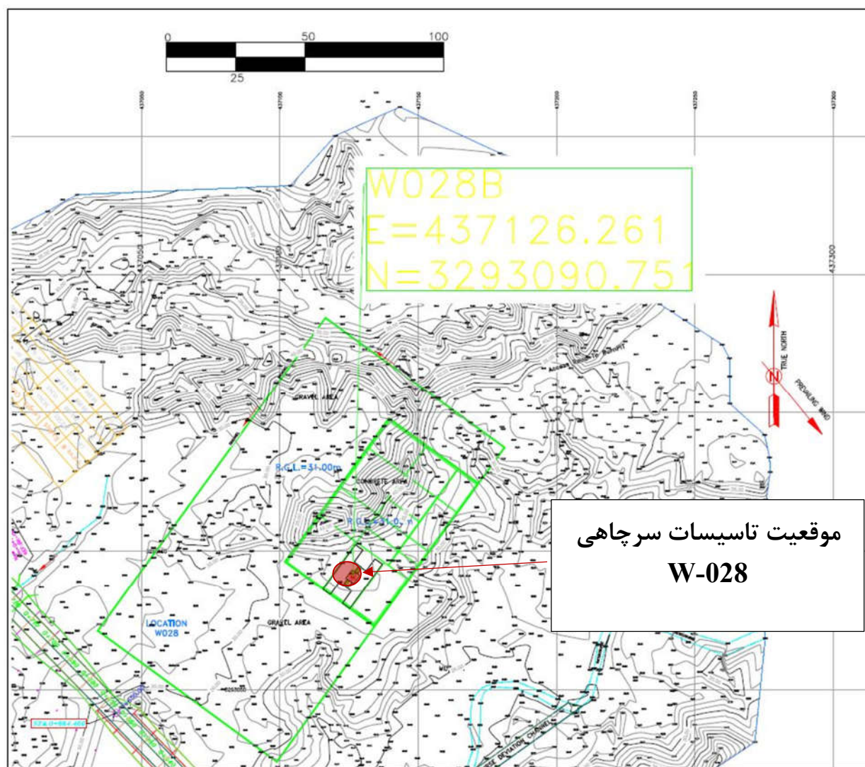
شکل 3-4. موقعیت قرارگیری تاسیسات سرچاهی در موقعیت W-018S در نقشه ارسالی از کارفرمای محترم
