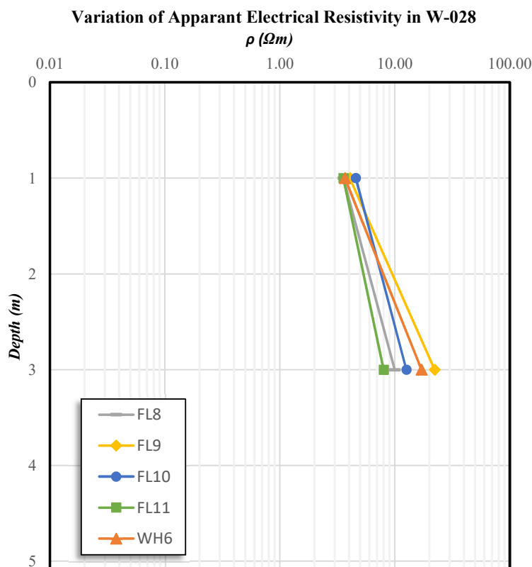
شکل 3-6- تغییرات مقاومت الکتریکی بر حسب عمق در مسیر خط لوله و تاسیسات سرچاهی بسته W-028
