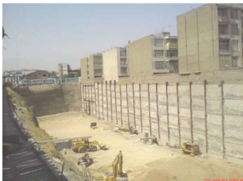
شکل 7-1 - تصاویری از سازه های نگهدارنده جهت گودبرداری (روش نیلینگ و دیوار برلنی)
