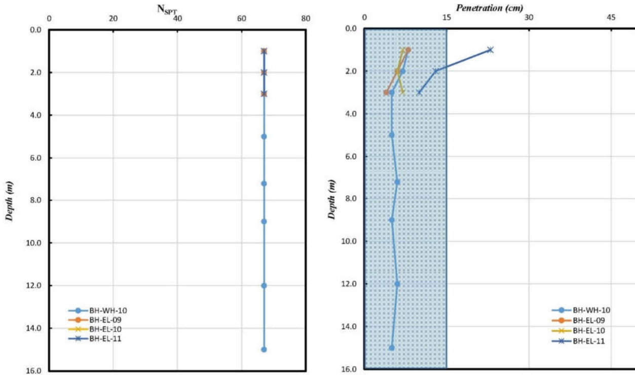
شکل 3-3- تغییرات نتایج ضربات SPT (اصلاح نشده) و میزان نفوذ متناظر بر حسب عمق بسته‌ی BK-14
