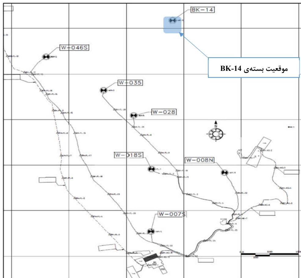
شکل 3-1- جانمایی محل حفر گمانه های ماشینی در موقعیت بسته ی BK-14 نسبت به مسیرهای خط لوله- نقشه ارسالی از شرکت محترم هیروگان انرژی
