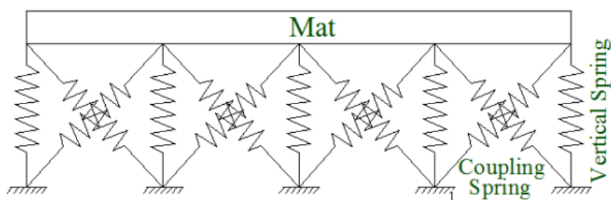
شکل ۶-۲. مدل سازی فنرهای کوپله
