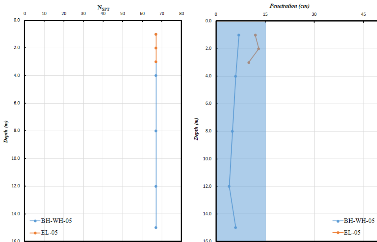
شکل ۳-۴- تغییرات نتایج ضربات SPT (اصلاح نشده) و میزان نفوذ متناظر برحسب عمق موقعیت بسته ی W-007S
