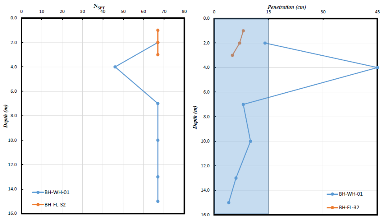
شکل ۳-۴- تغییرات نتایج ضربات SPT (اصلاح نشده) و میزان نفوذ متناظر برحسب عمق موقعیت بسته‌ی W-008N
