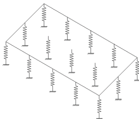
شکل ۶-۱. مدلسازی فنر وینکلر
