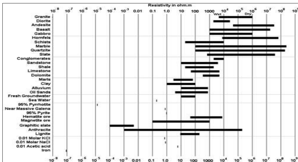
شکل ۳-۵- حدود مقاومت الکتریکی برای خاکهای مختلف
