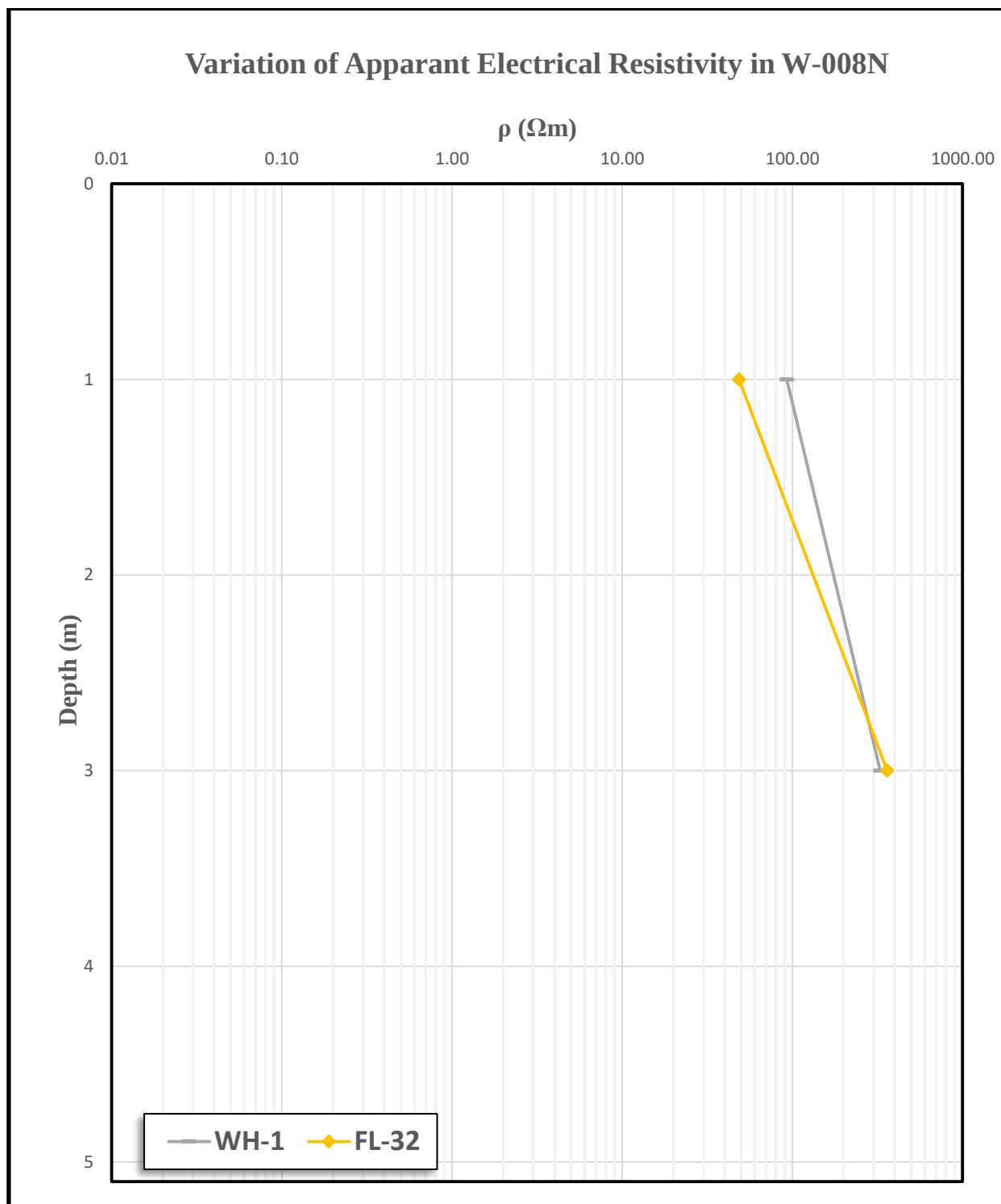
شکل ۳-۷- تغییرات مقاومت الکتریکی بر حسب عمق در موقعیت بسته‌ی W-008N
