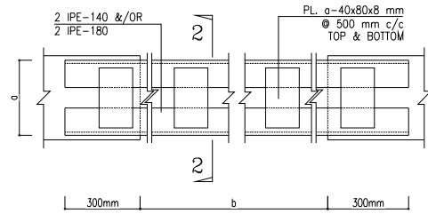
LINTEL PLAN -2 IPE Sc: N.T.S.
