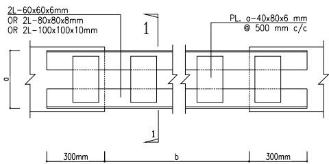
LINTEL PLAN -2L Sc: N.T.S.
