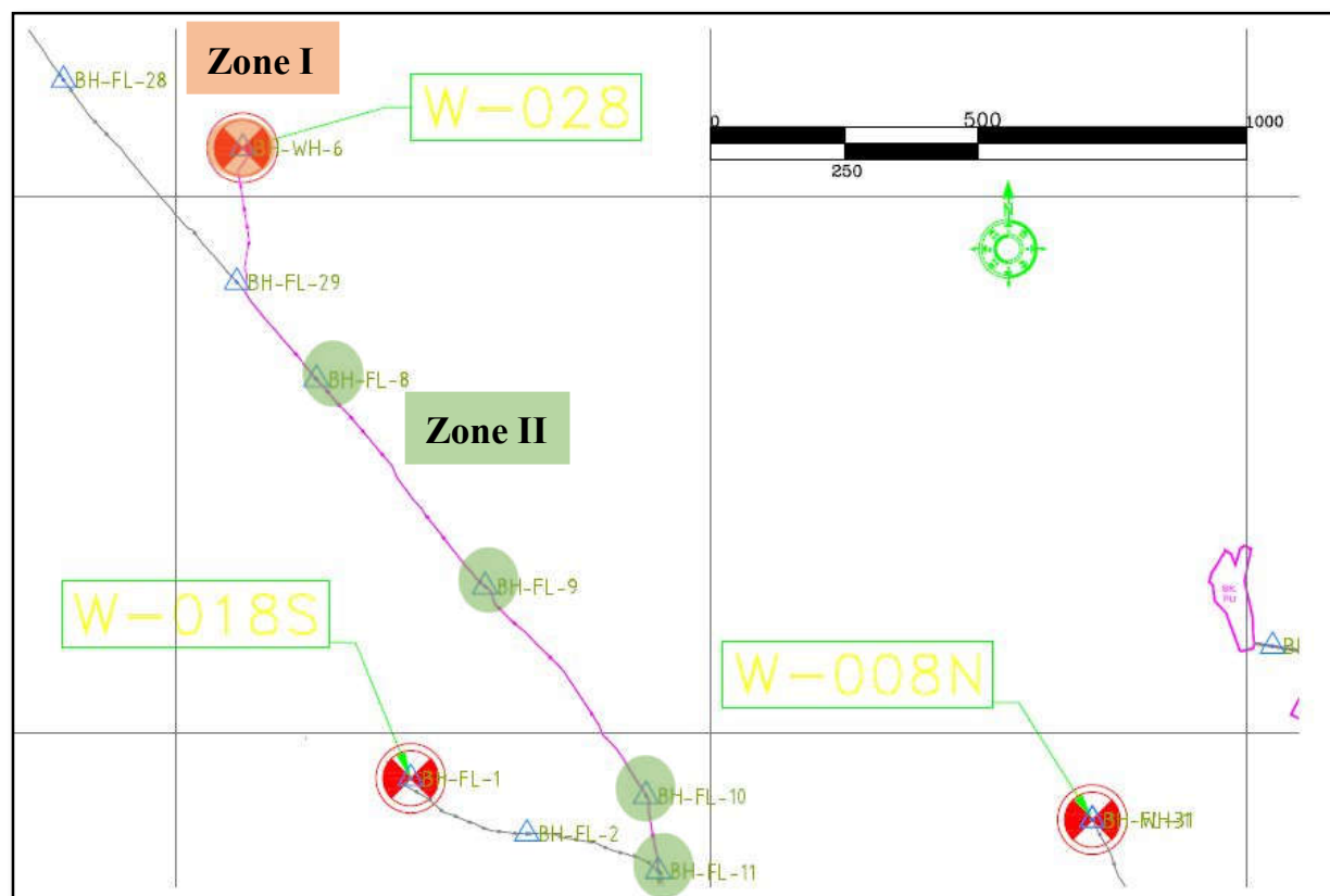
شکل 4-2. مرز تفکیکی زون های 1 و 2- نقشه ارسالی از کارفرمای محترم
