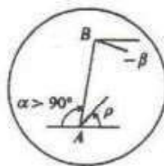
(a) گود گسیختگی مورد استفاده در روش Coulomb برای فشار محرک خاک
