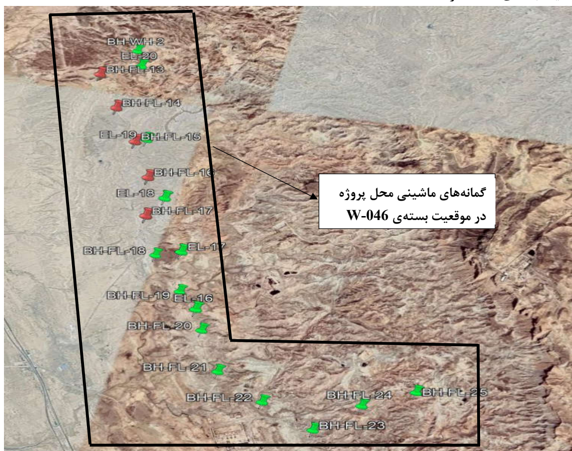
شکل 3-1- جانمایی محل حفر گمانه های ماشینی در موقعیت بسته ی W-046
