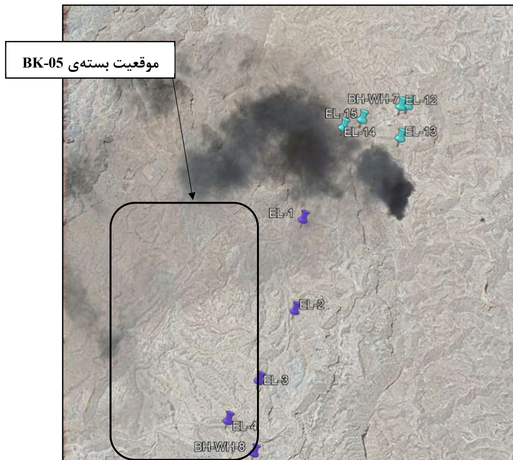
شکل 3-1- جانمایی محل حفر گمانه های ماشینی در موقعیت بسته ی BK-05
