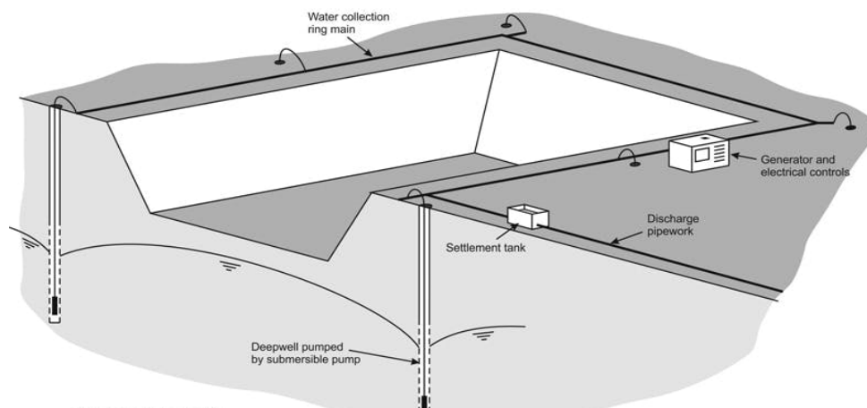
شکل 7-5 - سیستم آبکشی از چاه های عمیق
