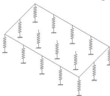
شکل 6-1- مدلسازی فنر وینکلر
