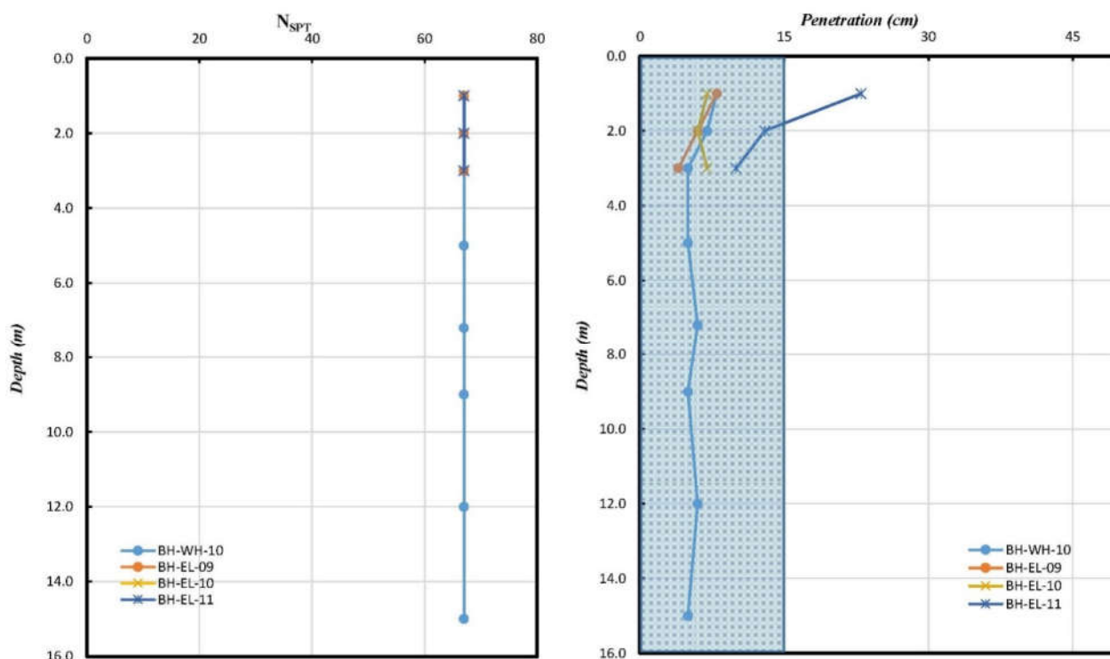
شکل 3-3- تغییرات نتایج ضربات SPT (اصلاح نشده) و میزان نفوذ متناظر برحسب عمق بسته ی BK-14
