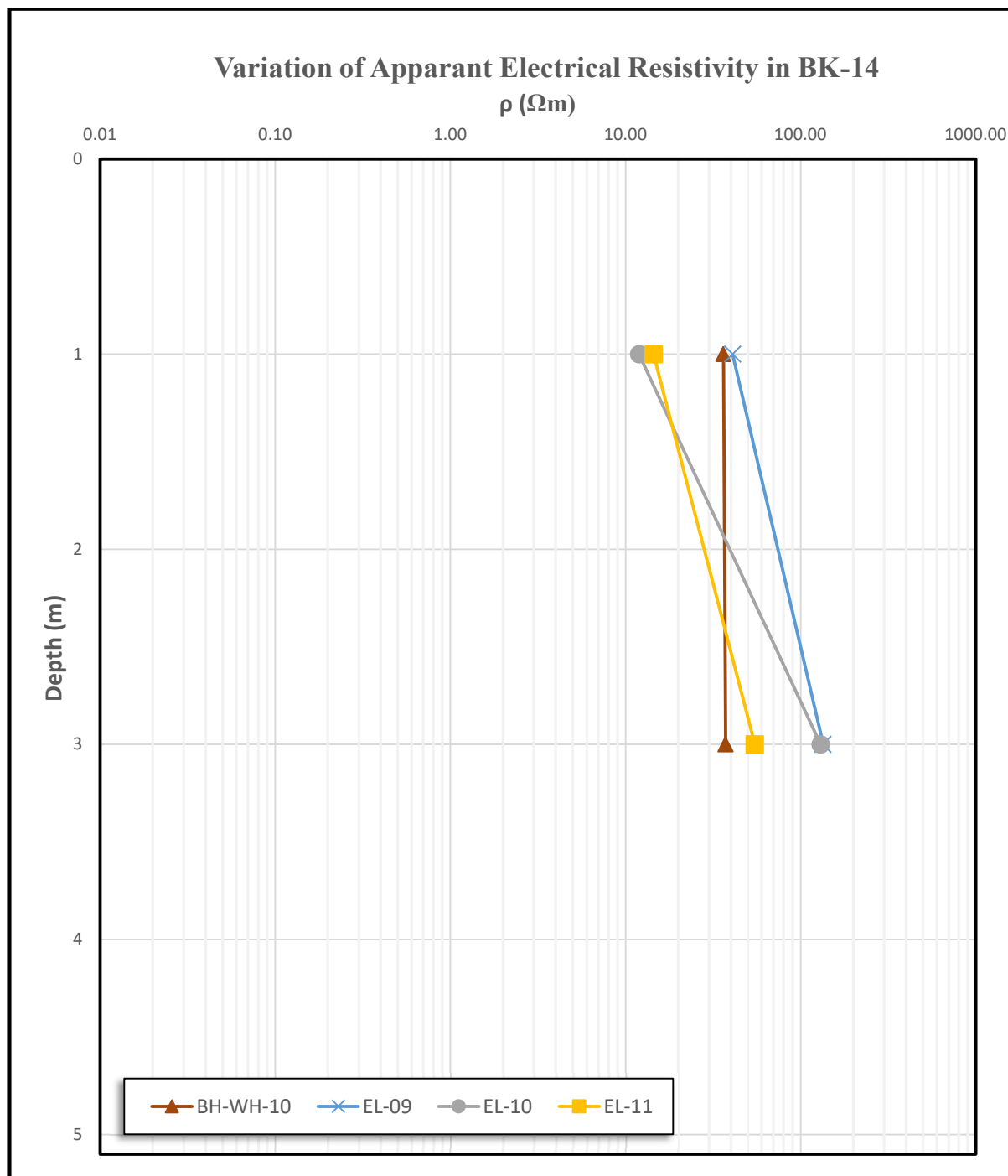
شکل 3-5- تغییرات مقاومت الکتریکی بر حسب عمق در بسته‌ی BK-14
