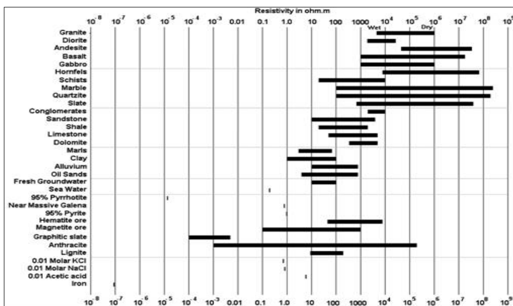
شکل 3-4- حدود مقاومت الکتریکی برای خاک های مختلف
