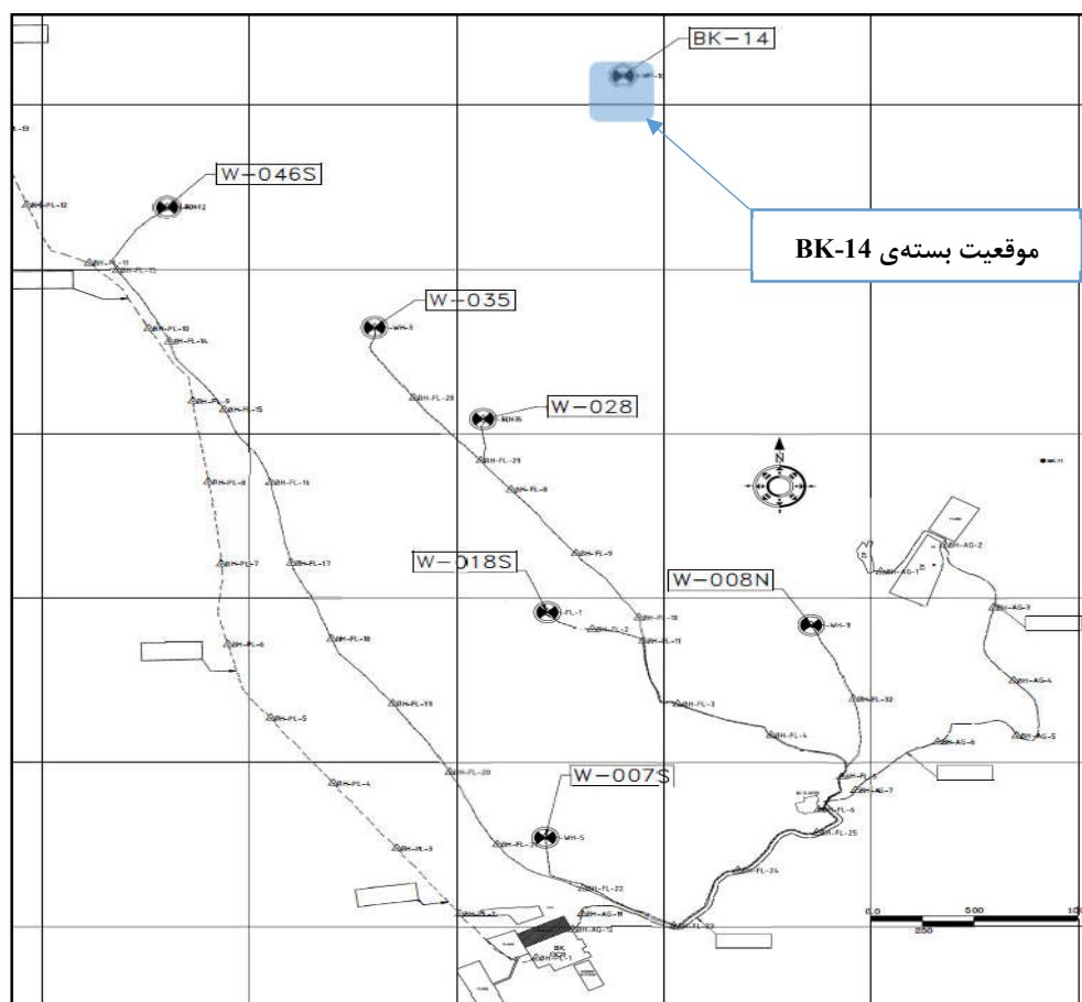
شکل 3-1- جانمایی محل حفر گمانه های ماشینی در موقعیت بسته ی BK-14 نسبت به مسیرهای خط لوله- نقشه ارسالی از شرکت محترم هیرگان انرژی
