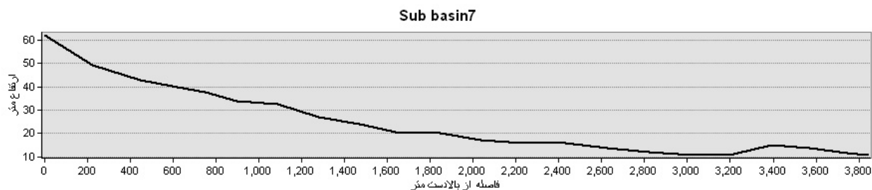
شکل 10-11- پروفیل طولی آبراهه در داخل حوضه آبریز در بردارنده سایت زیرحوضه 7
