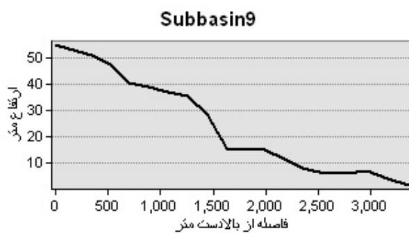
شکل 10-13- پروفیل طولی آبراهه در داخل حوضه آبریز در بردارنده سایت زیرحوضه 10 ایستگاه سرچاهی BK-05
