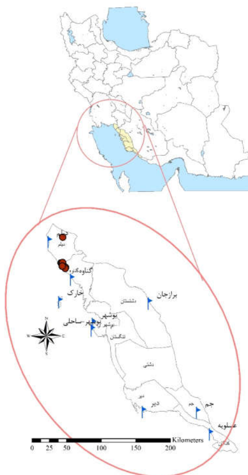
شکل 2-5 - موقعیت ایستگاه‌های سینوپتیک در استان بوشهر
