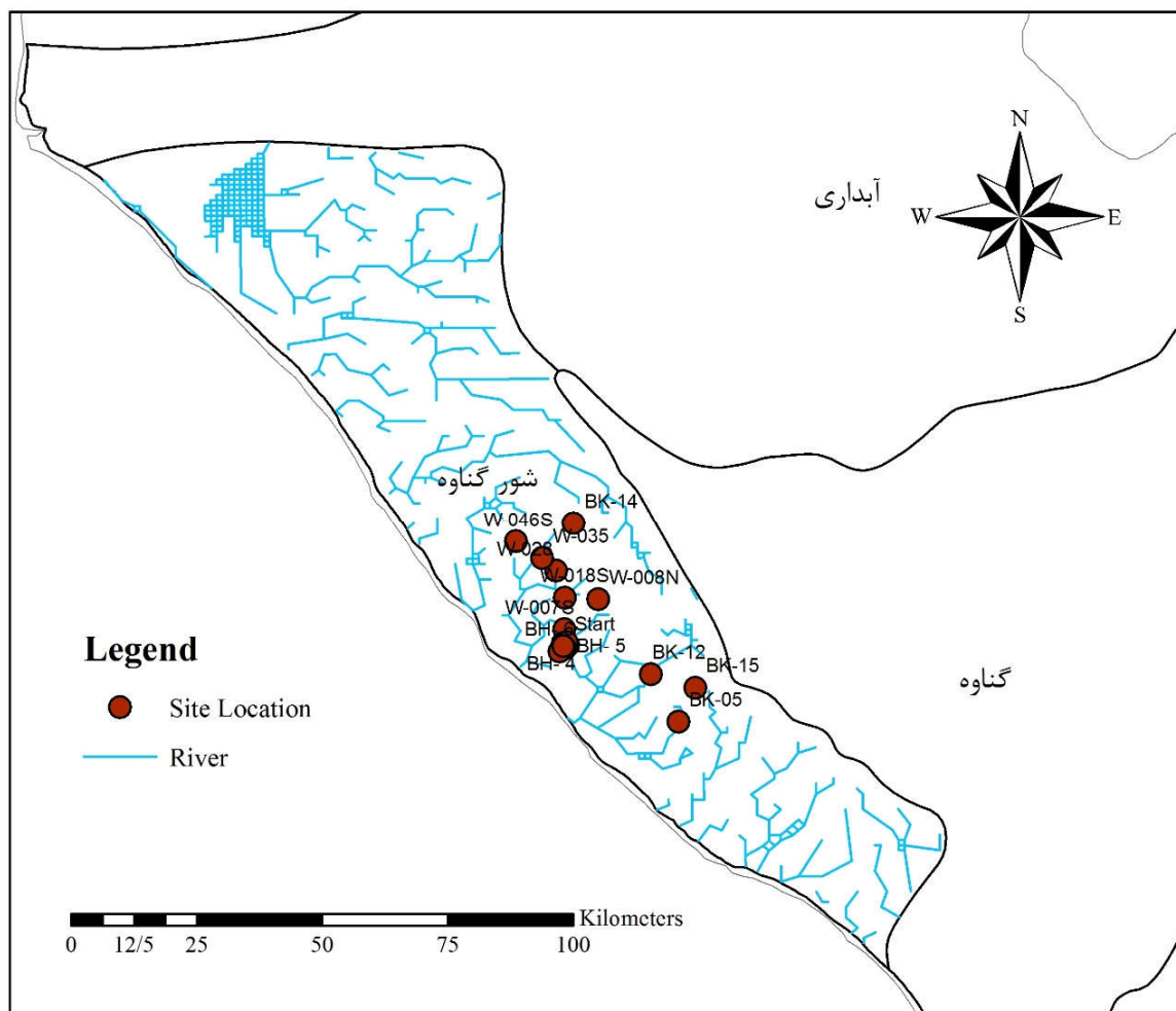
شکل 10-1 نقشه مسیرهای جریان‌های سطحی در زیر حوضه آبریز شور گناوه
