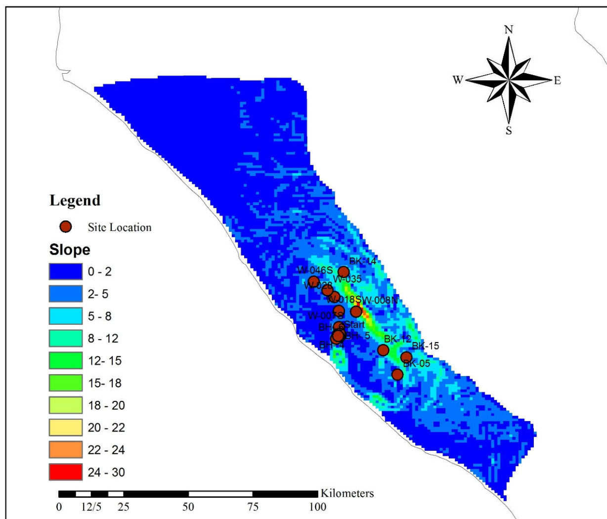
شکل 8-1- مدل شیب منطقه در زیر حوضه شور گناوه
