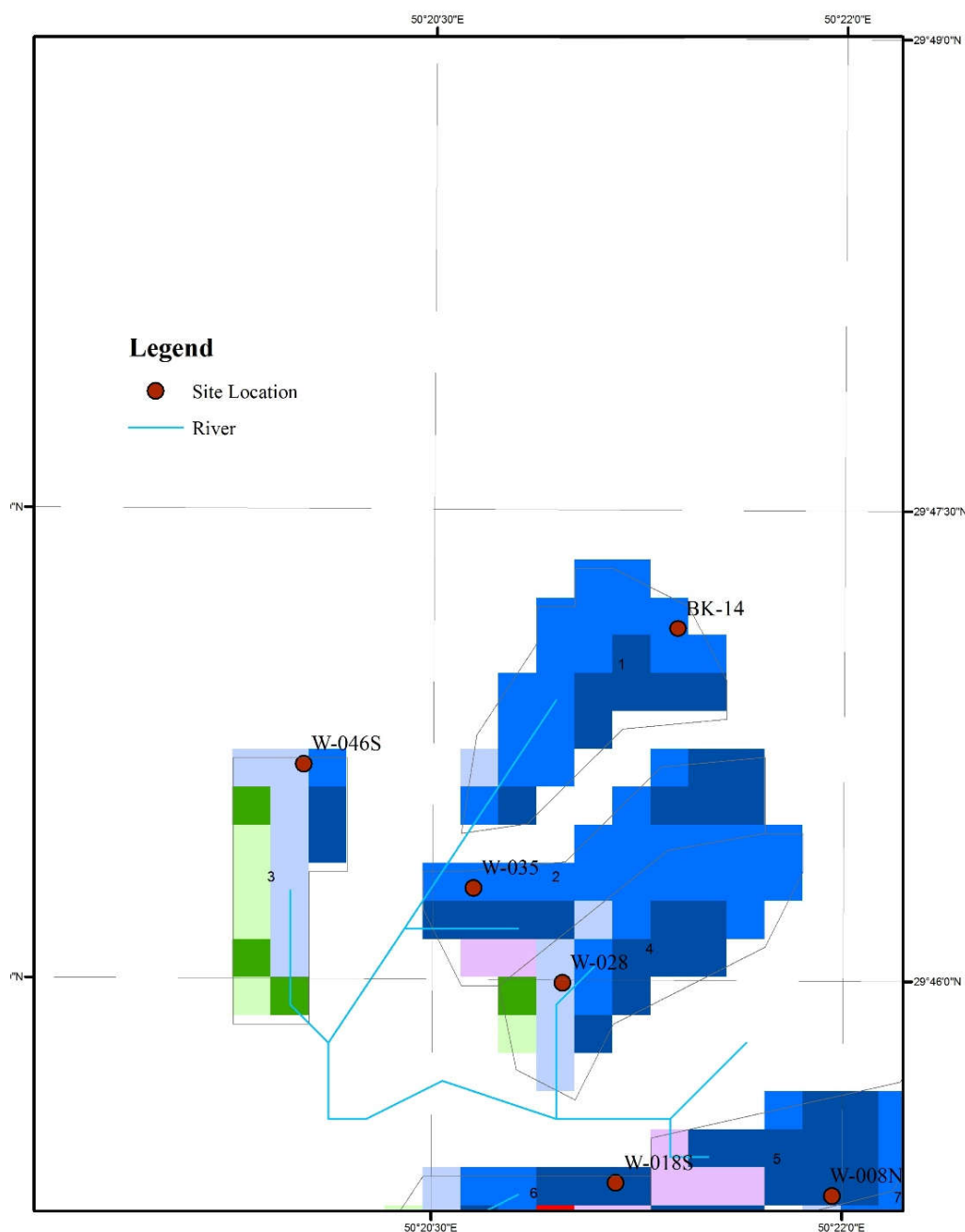
شکل 10-2- نقشه مسیرهای جریان‌های سطحی در زیر حوضه آبریز در بردارنده ایستگاه های سرچاهی W-046S و BK-14 و W-028 و W-035
