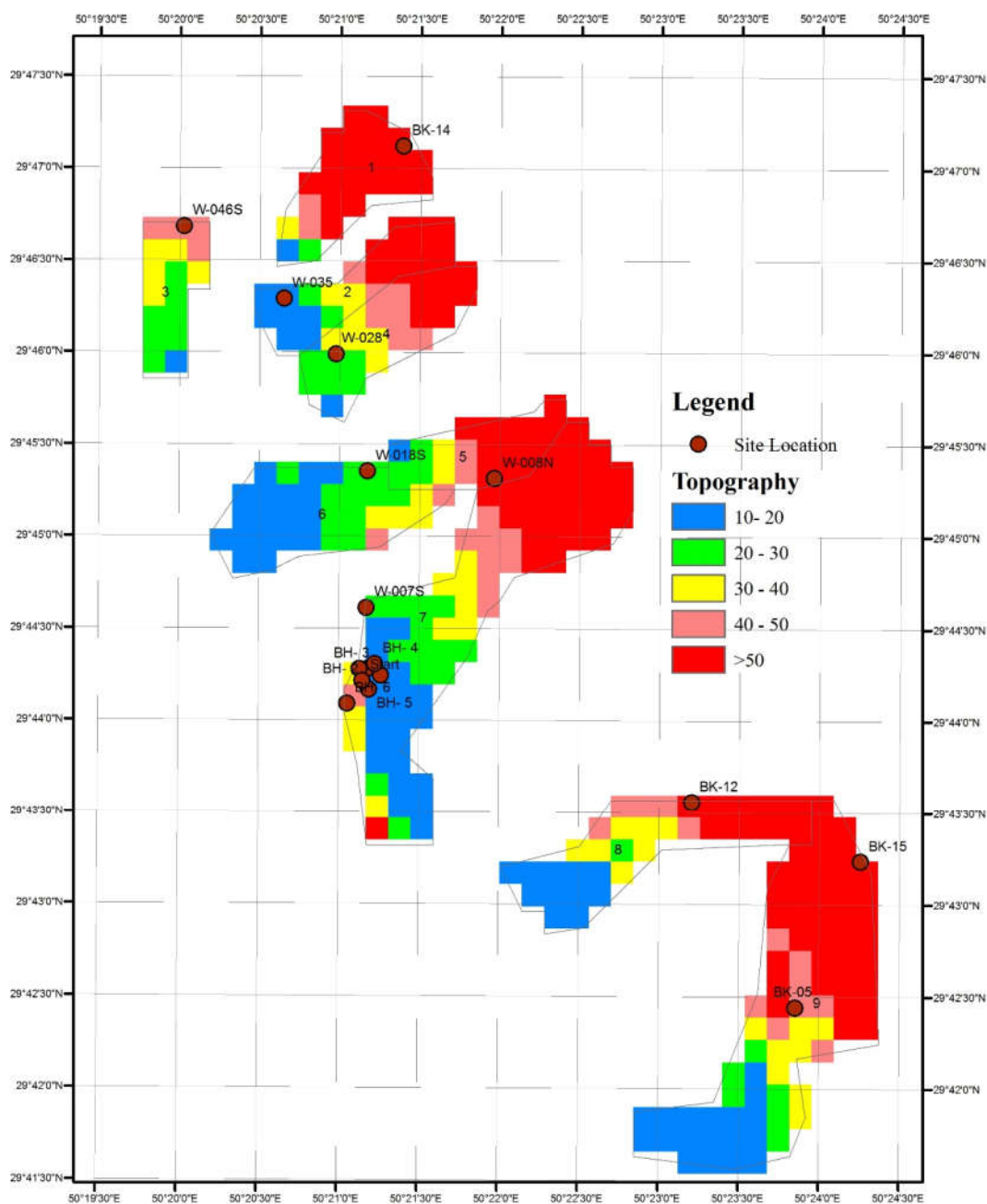
شکل 7-3 مدل ارتفاعی رقومی حوزه های آبریز در بردارنده سایت مورد مطالعه و ایستگاه های سرچاهی
