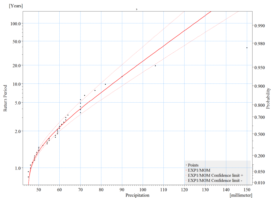
شکل 13-12- برازش توزیع آماری نمایی بر روی سری زمانی بلند مدت بارش روزانه در ایستگاه باران سنجی بی بی حکیمه
