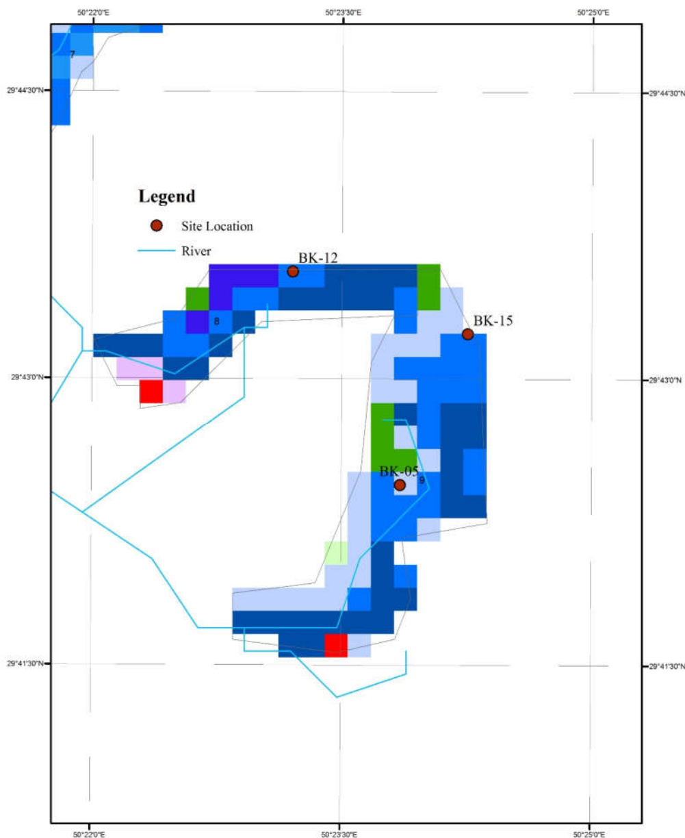
شکل 10-4 - نقشه مسیرهای جریان‌های سطحی در زیر حوضه آبریز در بردارنده ایستگاه‌های سرچاهی BK-12,15,5
