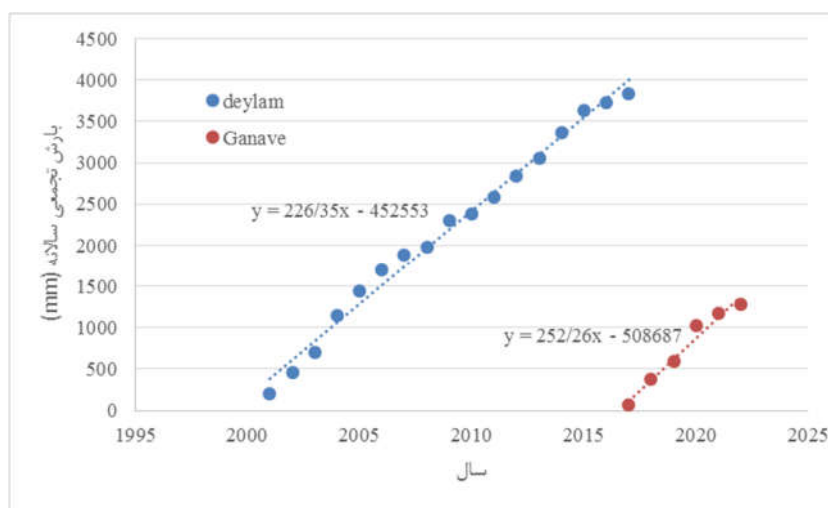
شکل 12-1- برازش خطی بر روی بارش تجمعی ایستگاه سینوپتیک دیلم و گناوه
