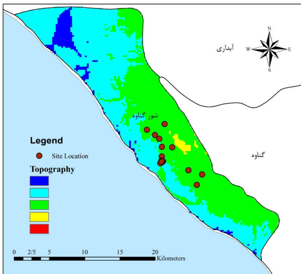
شکل 2-7- مدل ارتفاعی رقومی حوضه آبریز در شور گناوه
