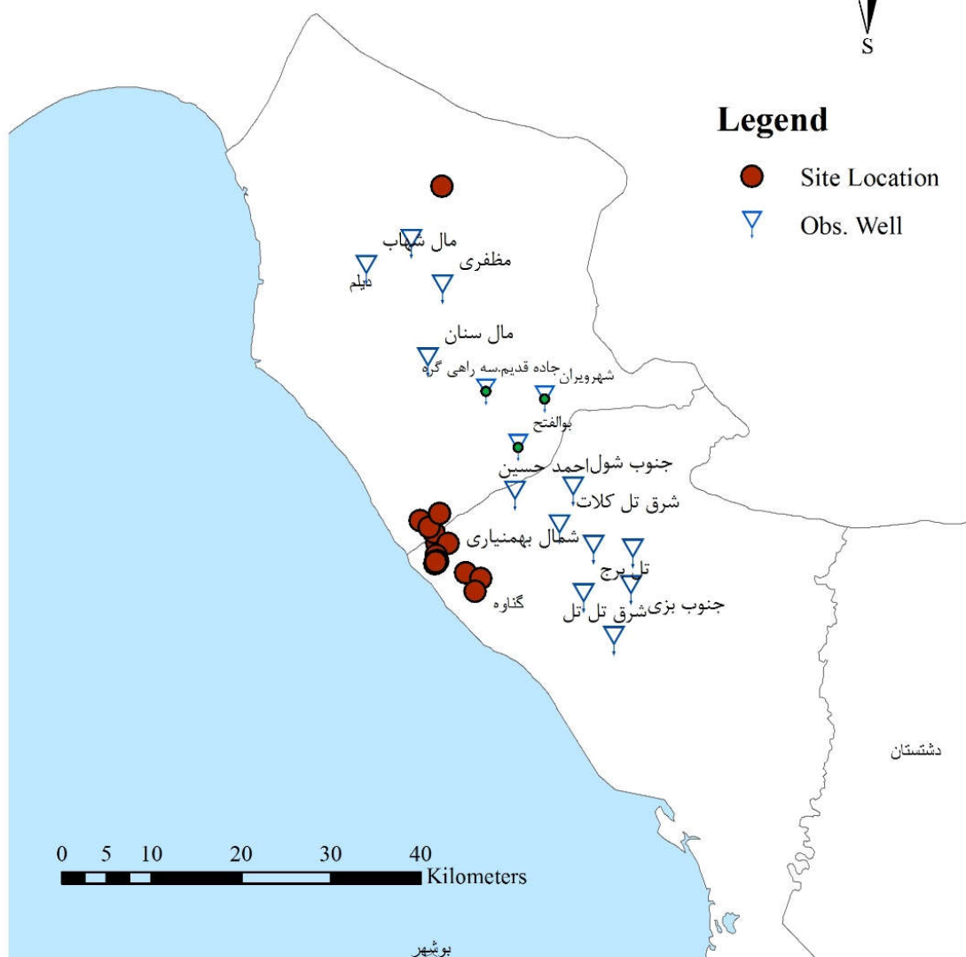
شکل 3-5- موقعیت ایستگاه‌های چاه مشاهداتی در اطراف سایت مورد مطالعه
