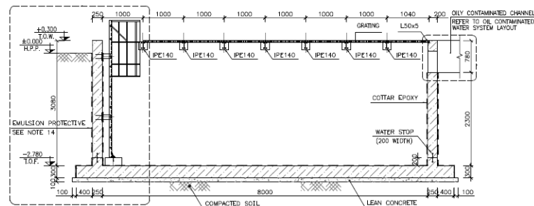
FIG 5 - Elevation View(SU-2201B)
