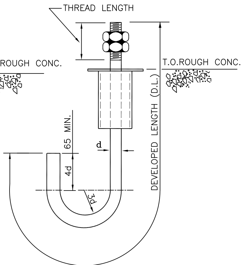
TYPE "JS"
