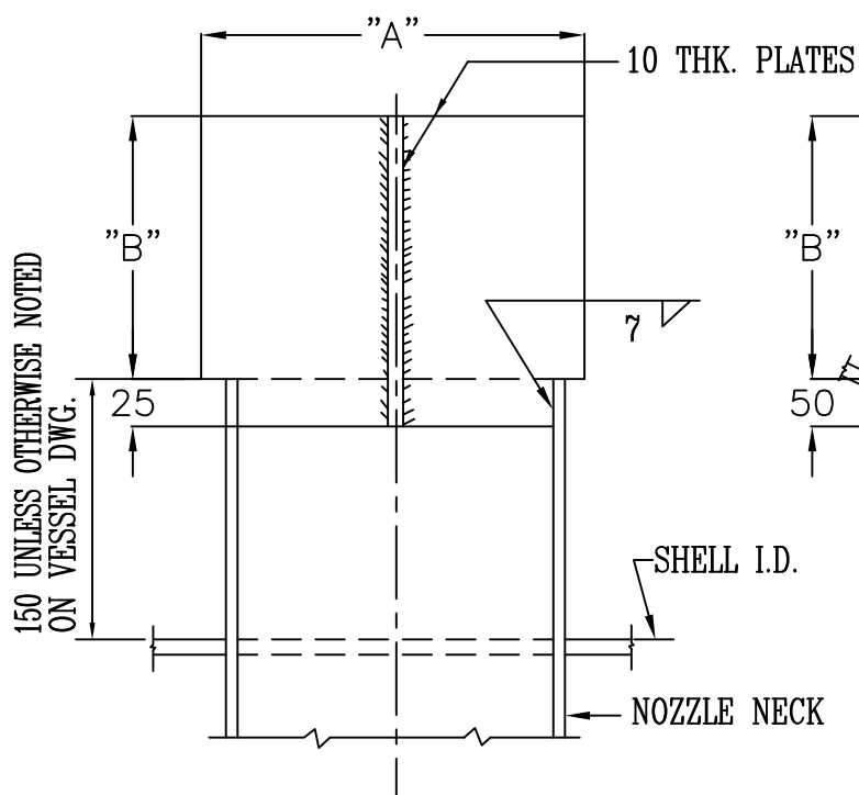
TYPE-A
