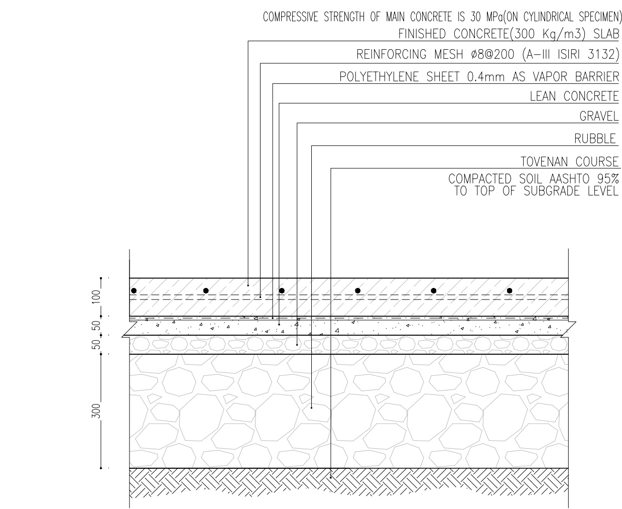
DETAIL 03 Sc:1/10
