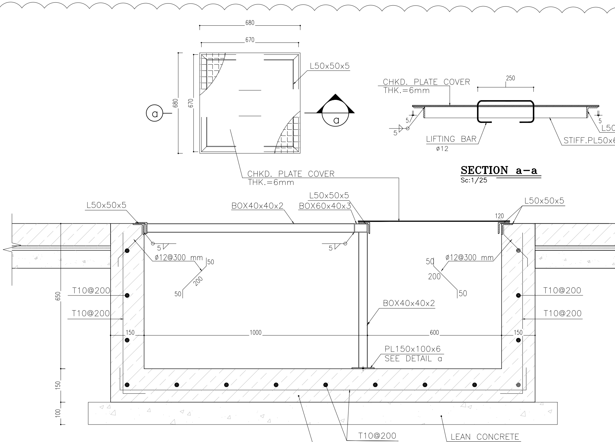
DETAIL 08 Sc:1/10
