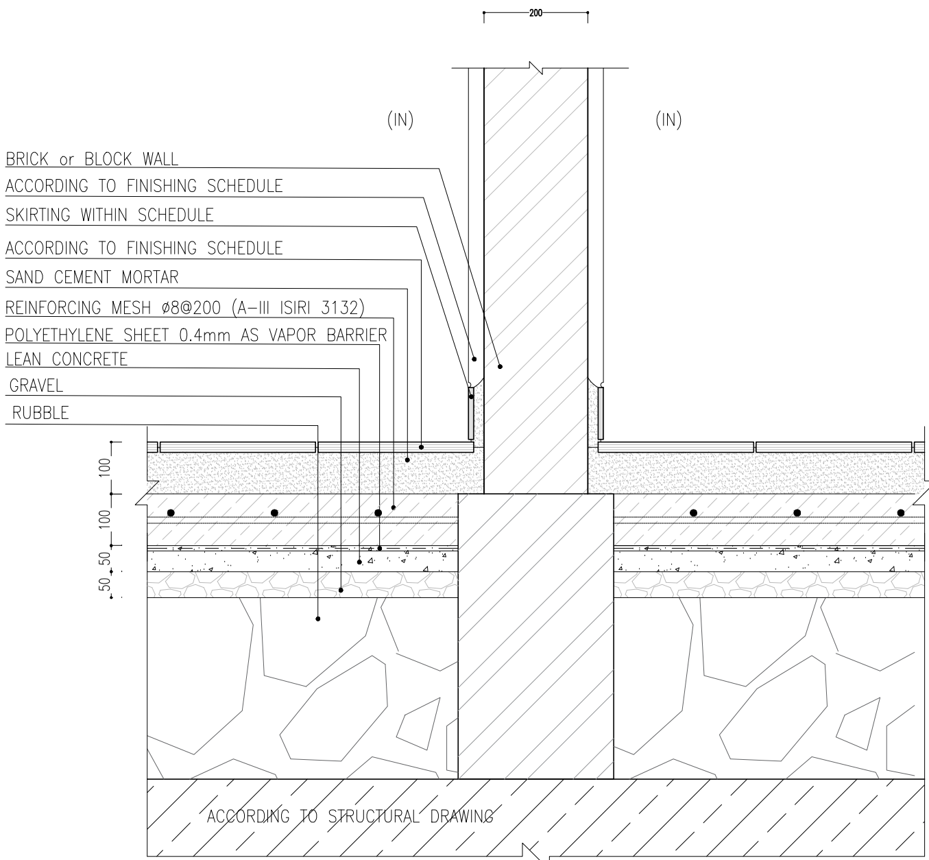
DETAIL 07 Sc:1/10
