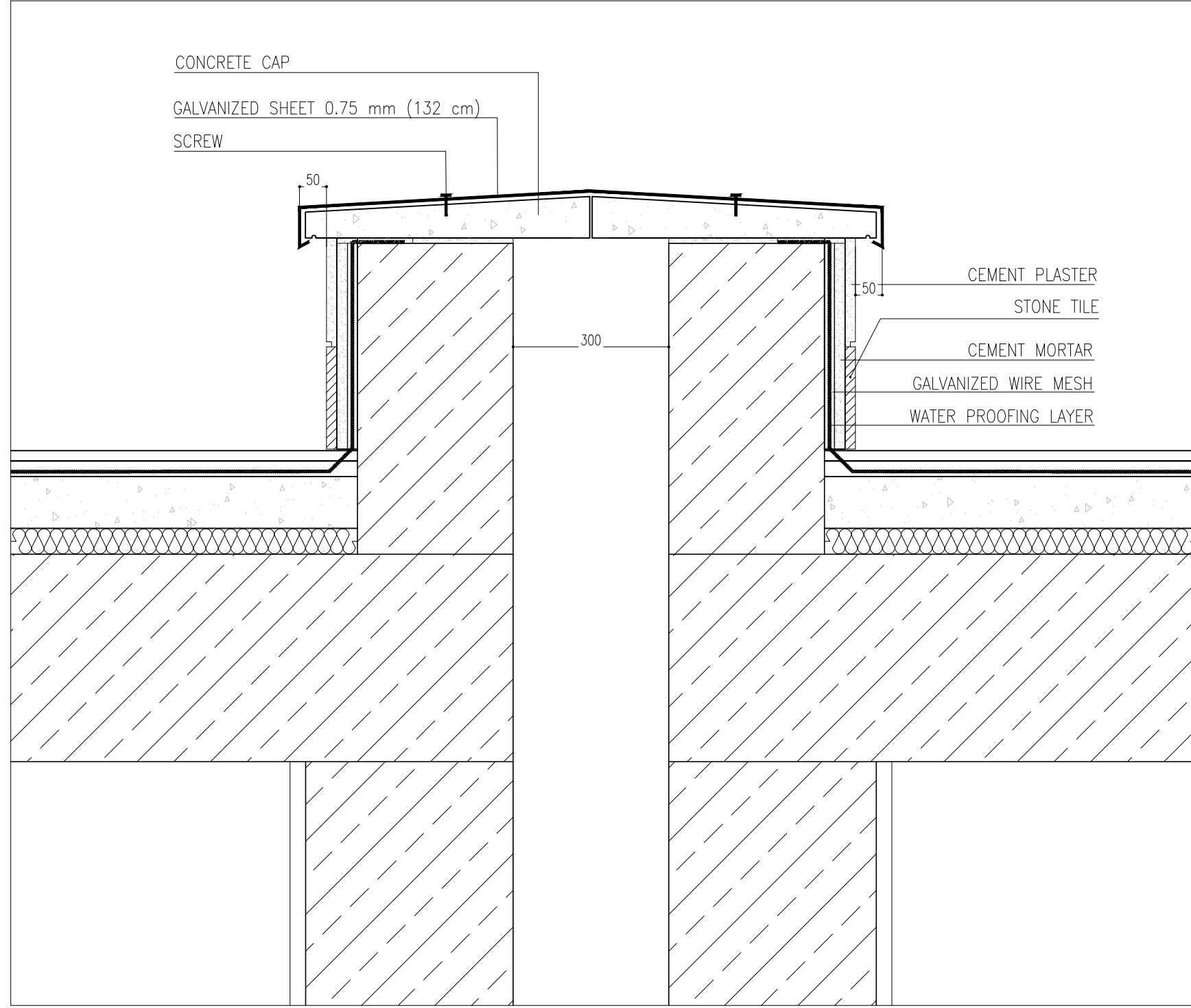
DETAIL 05 Sc:1/10
