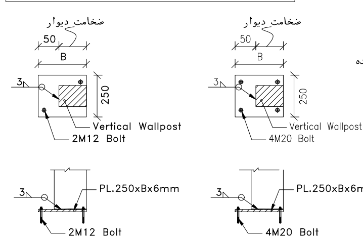
DETAIL-1a
