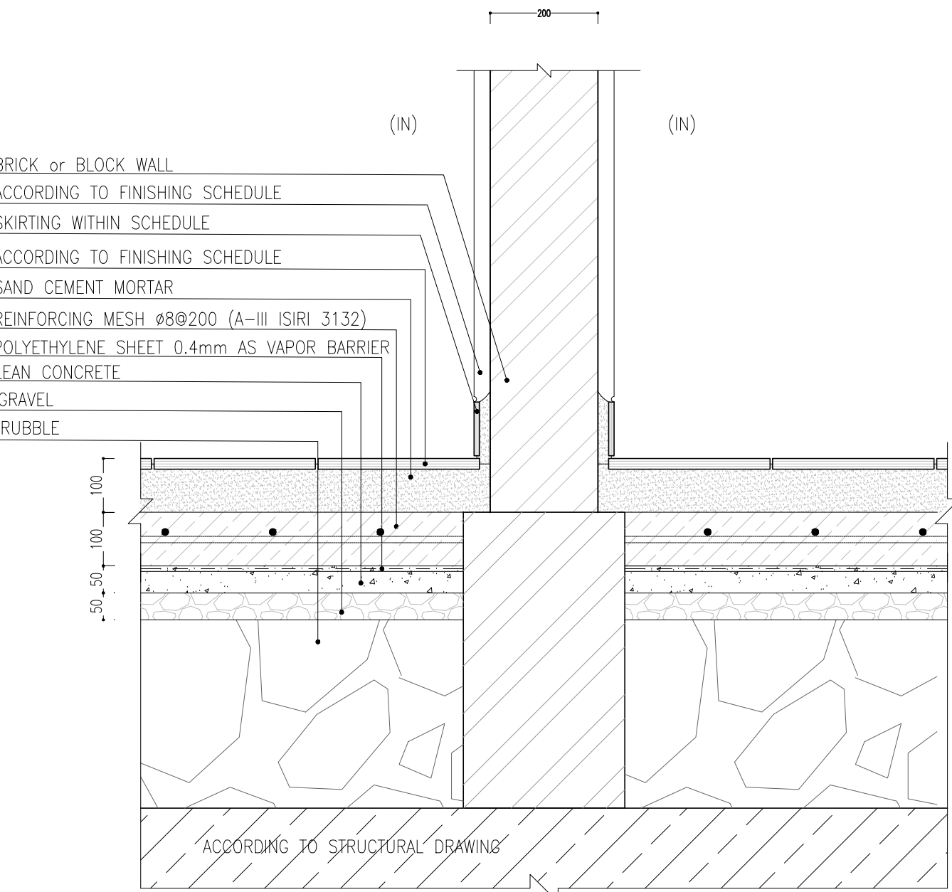
DETAIL 07 Sc:1/10
