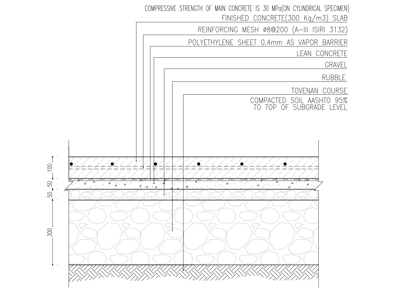
DETAIL 03 Sc:1/10
