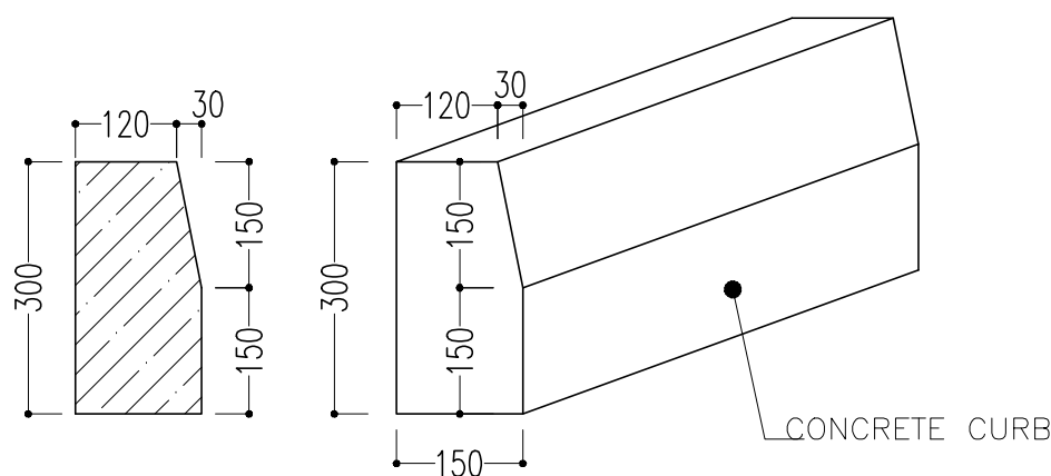
DETAIL 08 Sc:1/10
