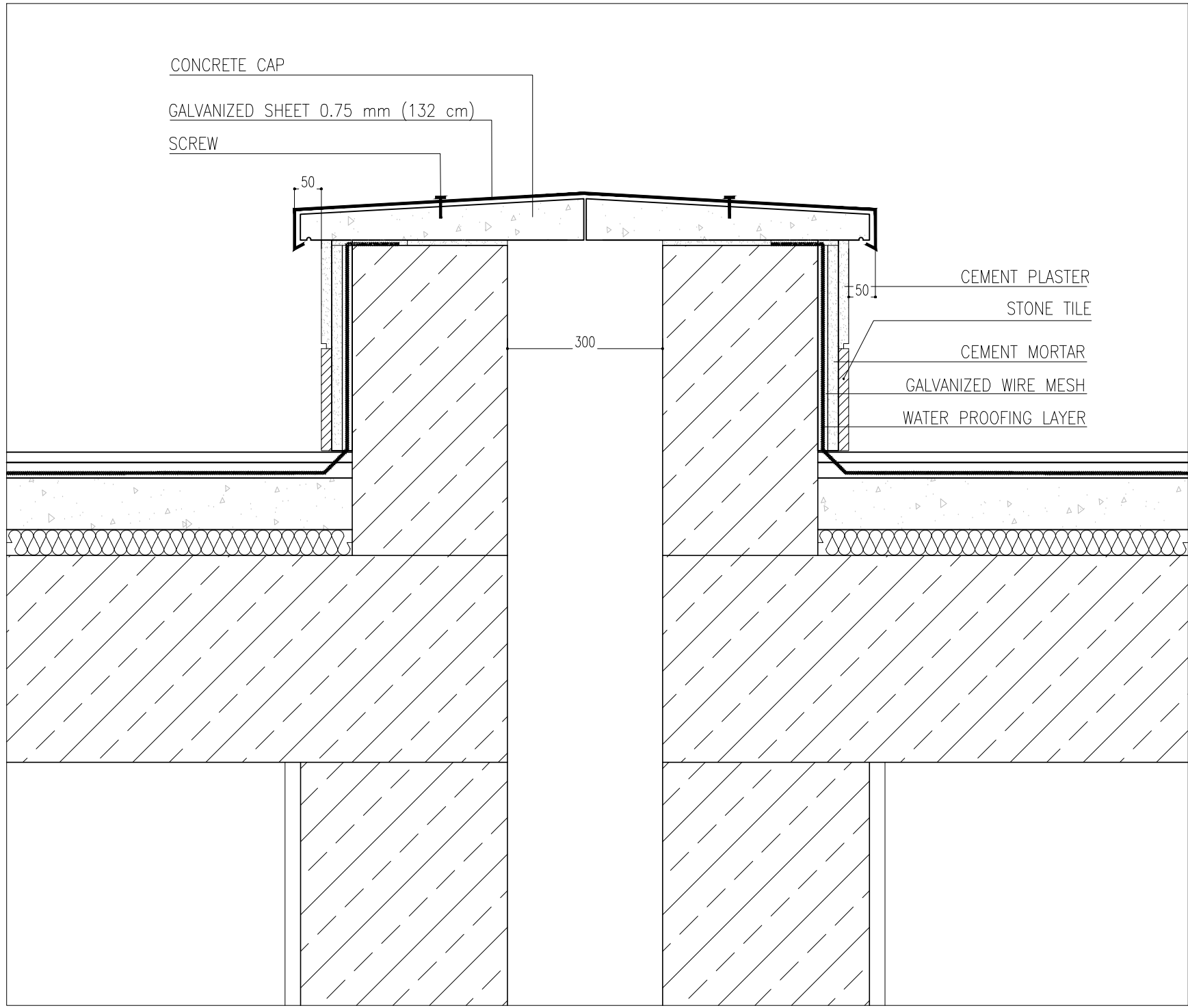
DETAIL 05 Sc:1/10
