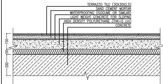
DETAIL 06 Sc:1/10
