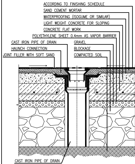
DETAIL 05 Sc:1/10
