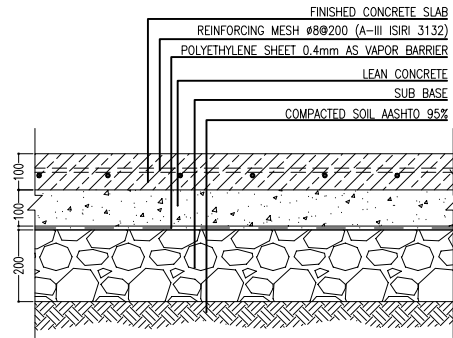
DETAIL 08 Sc:1/10
