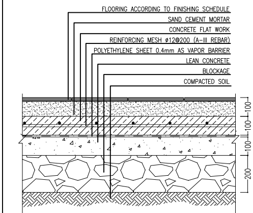
DETAIL 07 Sc:1/10
